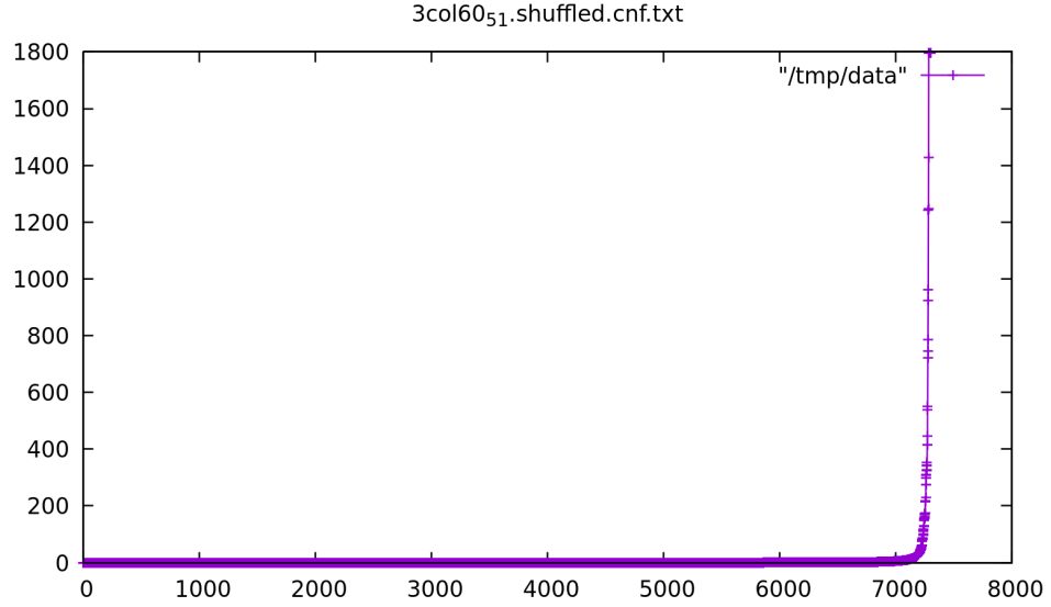
FIGURE 4.12 – Graphe représentant les temps des appels au Glasgow Subgraph Solver triés dans l'ordre croissant lorsque les isomorphismes étendus sont utilisés sur l'instance 3col60_5_1.cnf .
