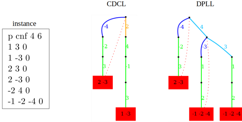
FIGURE 1.4 – Exemple d'arbre de recherche pour l'approche CDCL sur une instance incohérente. L'arbre de recherche pour l'approche DPLL avec la même heuristique est ensuite donné à titre de comparaison.
