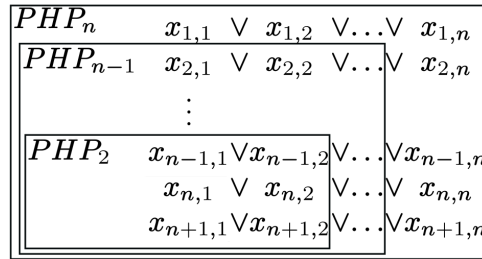
FIGURE 4.1 – Imbrication des sous-problèmes pour un problème de pigeons de taille n .
