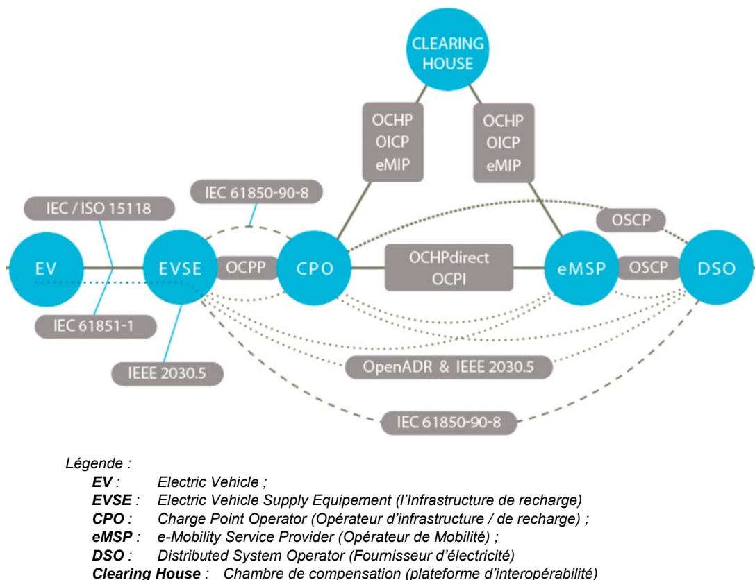
Figure 48 : Une recharge sans frontière : les standards de communication nécessaires.
