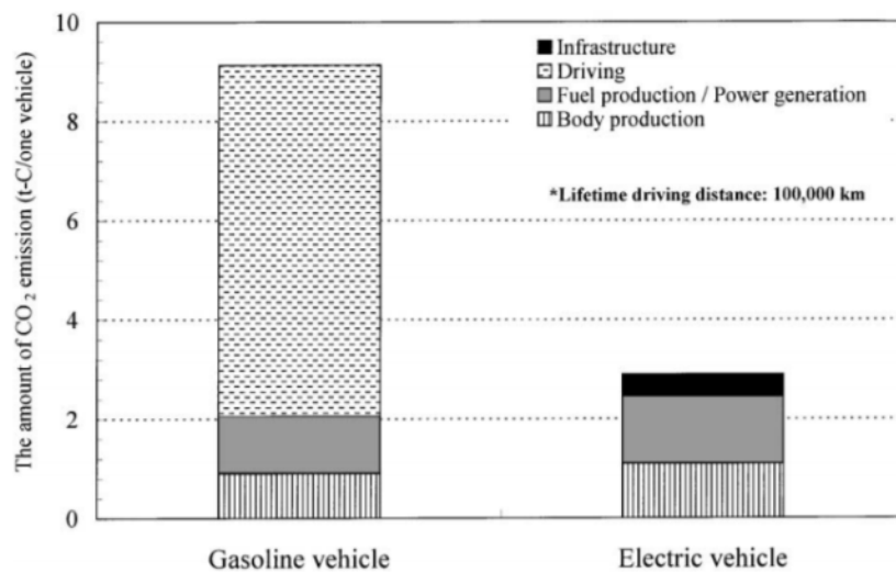
Figure 10 : Comparaison des émissions de CO 2 entre un véhicule thermique (Gasoline vehicle) et un véhicule électrique.
