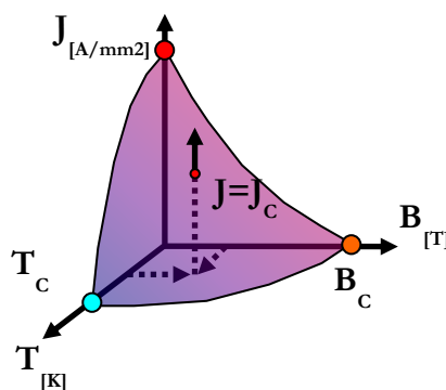
Figure 1. Surface critique d'existence de l'état supraconducteur.
