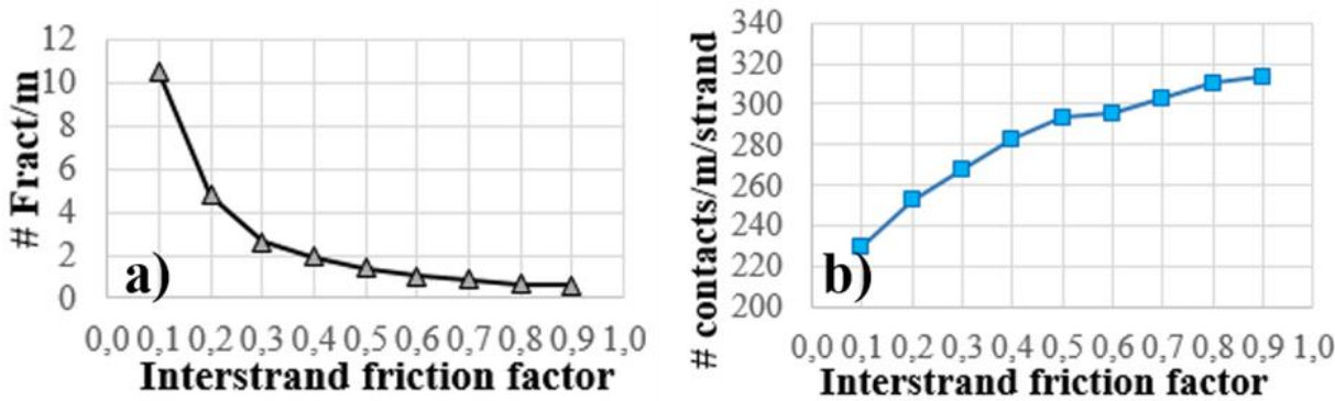
Figure 29. a) Variation du nombre de fractures par mètre en fonction du coefficient de frottement après CD. b) Variation du nombre de contacts par mètre et brin en fonction du coefficient de frottement après CD.
