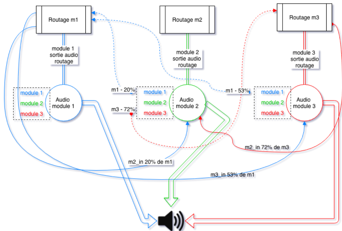
Figure 9 — Système de routage du signal audio entre modules
