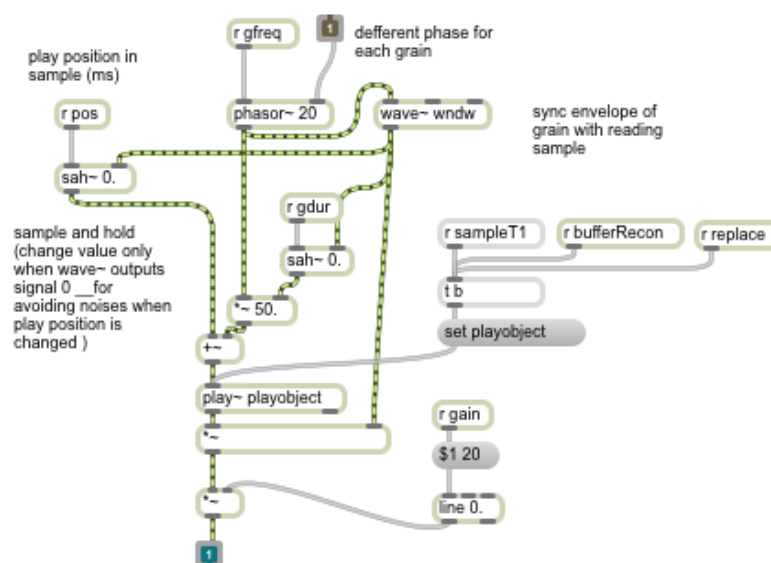
Figure 13 - Le moteur sonore de la synthèse granulaire
