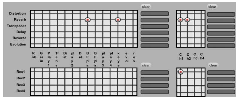
Figure 90 – Routage du signal sonore dans l'improvisation d' Unmapped
