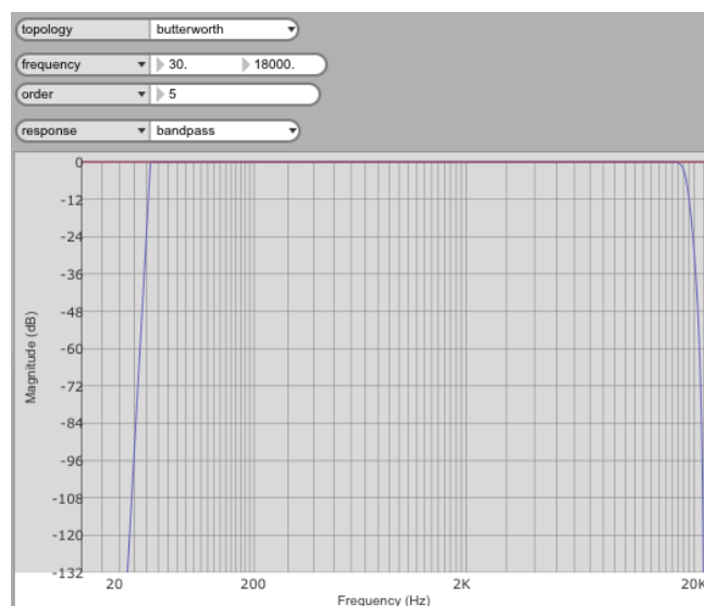
Figure 59 — Module de filtre générale 638 appliqué au son globale
