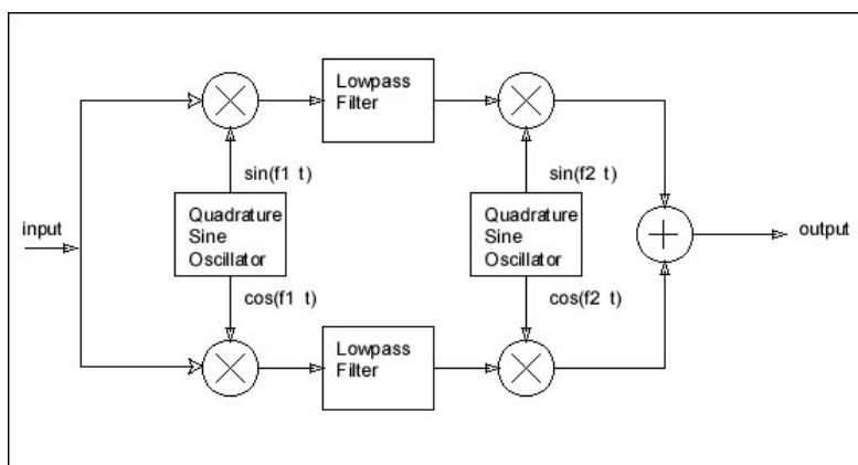
Figure 67 – Diagramme pour la transposition de fréquence 651
