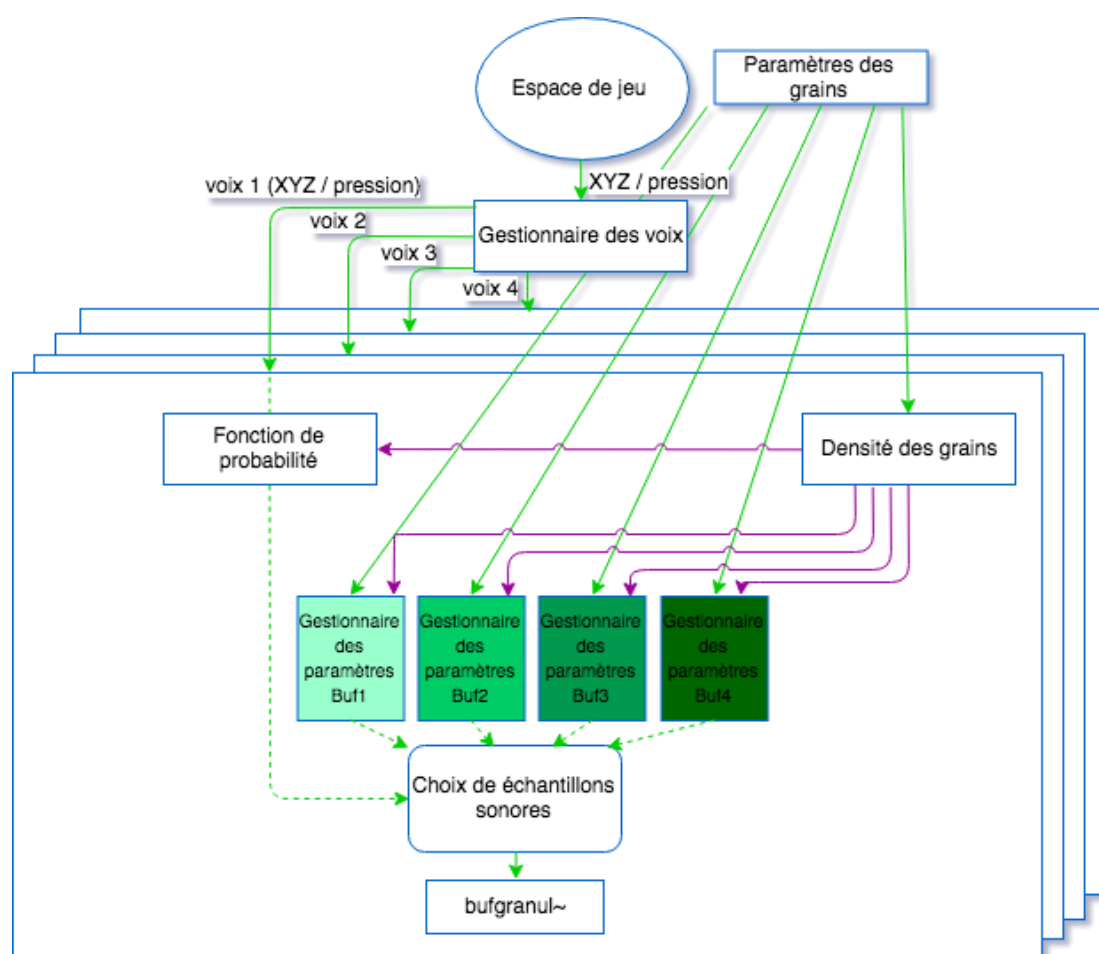
Figure 51 — Schéma du moteur sonore de Granulator .
