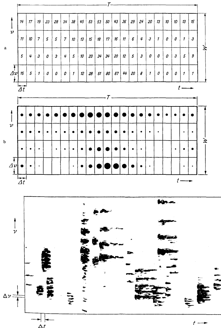
Figure 42 — Matrice de Gabor 575 .
