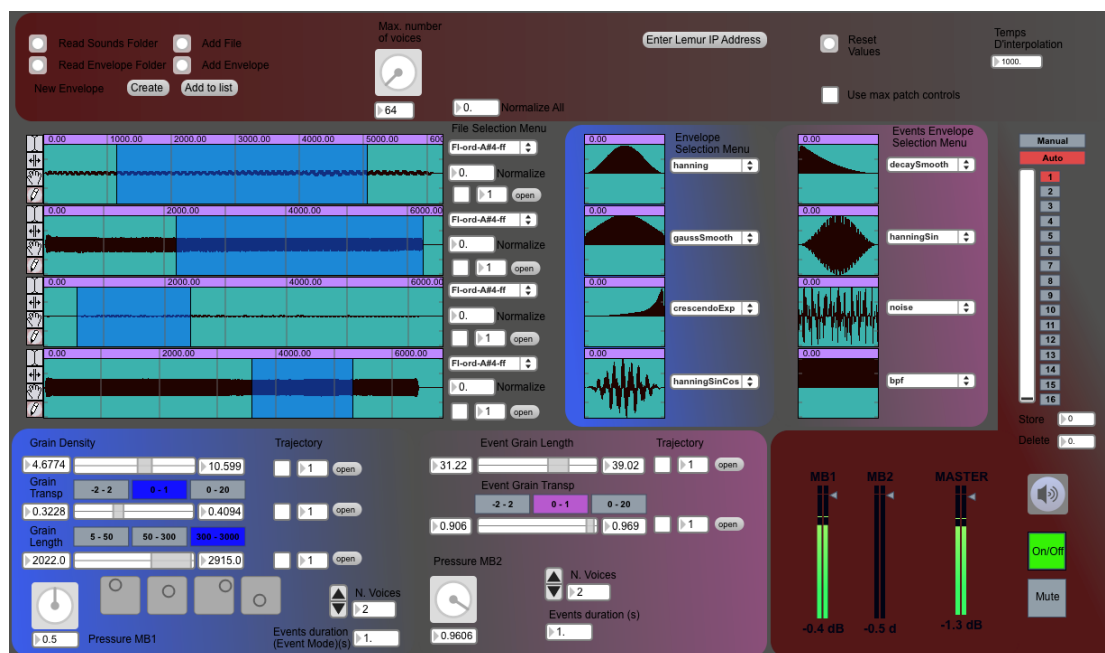
Figure 49 – Interface utilisateur du moteur sonore sur Max/MSP
