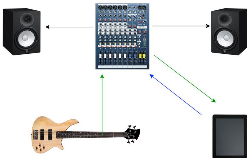
Figure 91 – Configuration audionumérique pour l'improvisation Reload de Electrologues .
