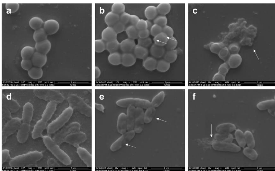
Figure 65: Images MEB de S. aureus non traitée (a), S. aureus exposée à la thymoquinone à une concentration égale à la CMI (b), S. aureus exposée à la thymoquinone à une concentration égale à 2xCMI (c), E. coli non traitée (d), E. coli exposée à la thymoquinone à une concentration égale à la CMI (e), E. coli exposée à la thymoquinone à une concentration égale à 2xCMI (f) [125]
