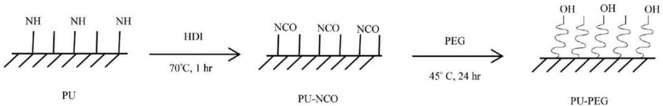
Figure 20: Greffage de polyéthylène glycol (PEG) sur une surface de polyuréthane (PU) en utilisant l'hexaméthylène diisocyanate (HDI) comme agent de couplage [61]
