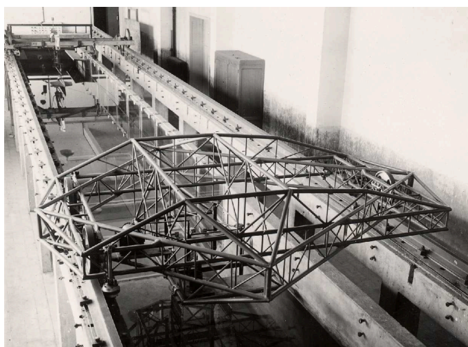
FIGURE 2.7 – Canal hydrodynamique [Archives de l'ONERA Lille].
