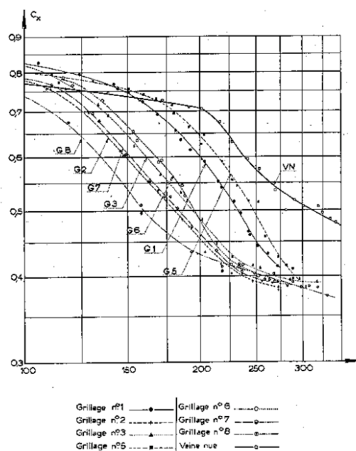
FIGURE 3.6 – Réseau de courbes C_x en fonction du nombre de Reynolds, avec différents grillages pour une sphère de diamètre de 80 mm (a) et un cylindre de diamètre 88 mm (b). La comparaison des résultats montre que la courbe relative au cylindre présente un caractère de régularité plus marqué par rapport à la courbe obtenue au moyen de la sphère [Guienne 1940].
