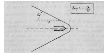
FIGURE 1.9 – Une onde balistique à grande vitesse [Darrieus 1922, 242].
