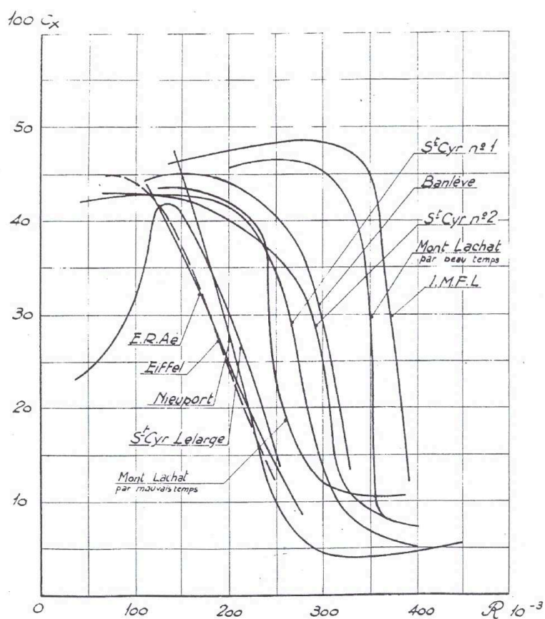
FIGURE 5.3 – Comparaison des divers nombres critiques de Reynolds en fonction du coefficient de traînée obtenus dans une dizaine de soufflerie. Nous pouvons remarquer la valeur 370000 correspondant à l'IMFL, ce qui indique une turbulence très faible par rapport aux autres [Moraux 1943].
