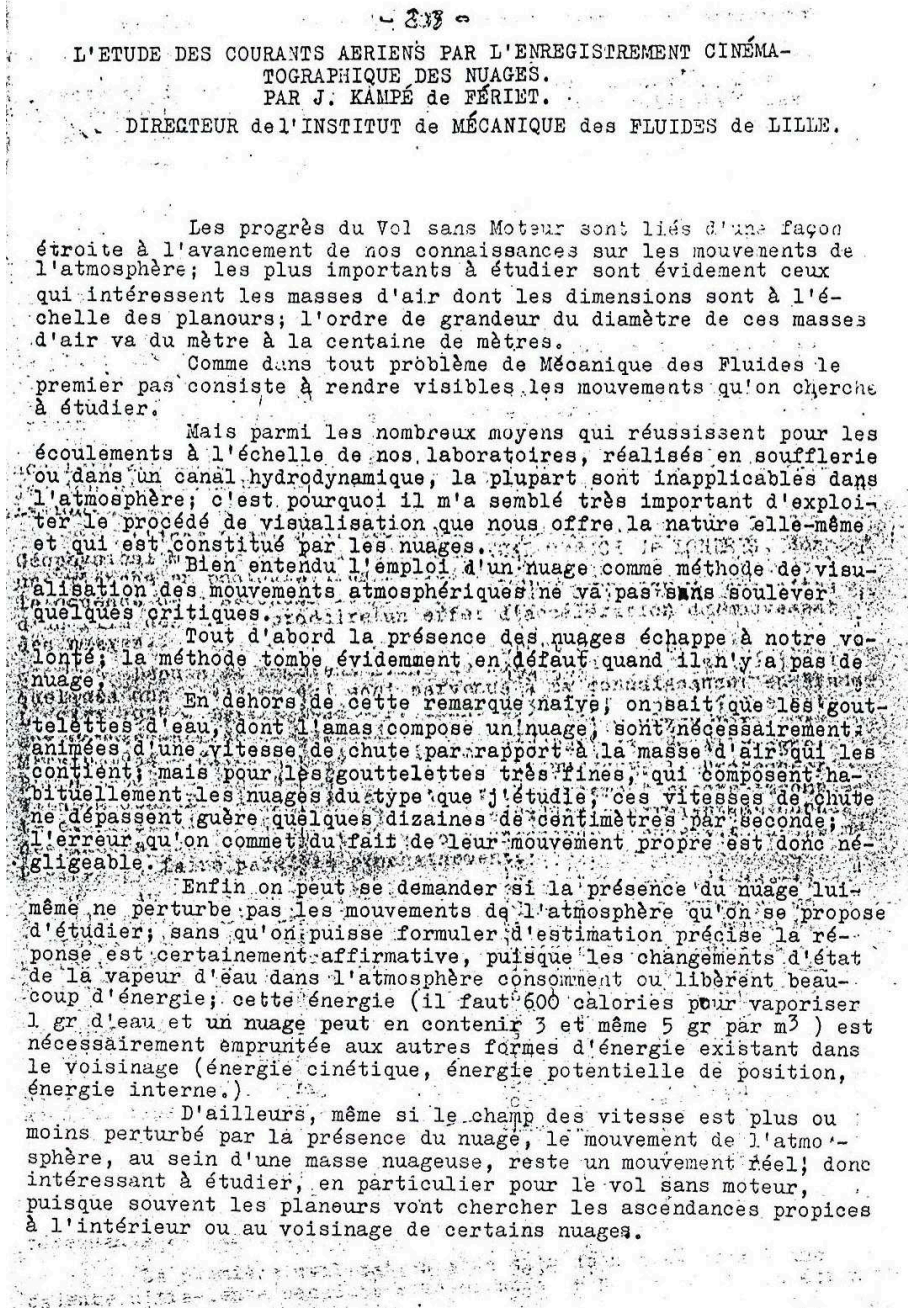
FIGURE A.1 – Les travaux expérimentaux de Kampé de Fériet, p. 1
