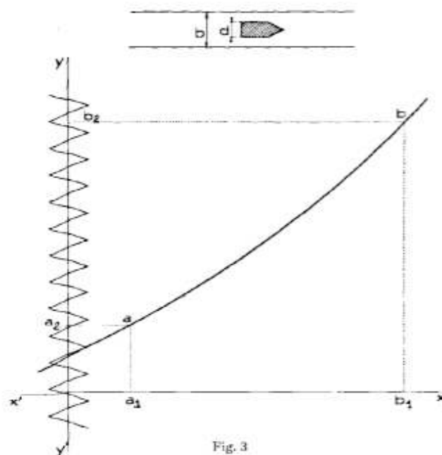
FIGURE 1.11 – Le mouvement relatif de l'image du projectile sur une plaque en mouvement [Vagner 1937, 36].
