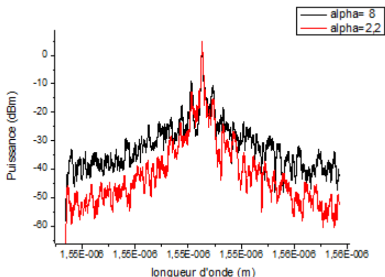
Figure IV. 26. Spectre du signal en sortie du DML-TR (pour \alpha=8, 2.2 ).
