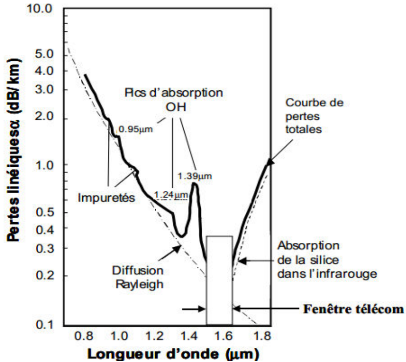
Figure II. 2 Courbe schématisée des pertes par atténuation en fonction de la longueur d'onde dans une fibre optique standard [21].
