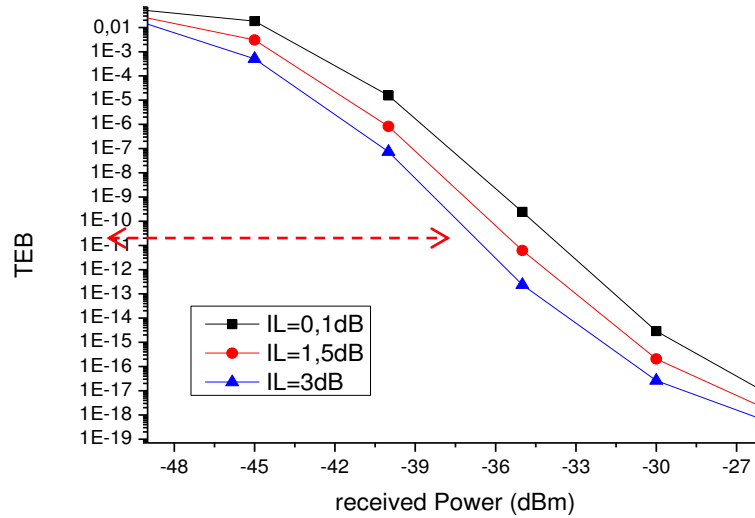
Figure IV. 13 TEB en fonction de la puissance à l'entrée du démux pour différentes valeurs de IL.
