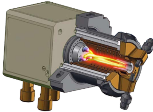
Figure 21 : Coupe schématisique de la torche TriplexPro-200 (d'après Sulzer Metco)
