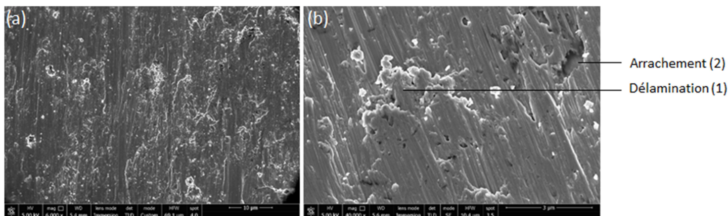
Figure 98 : Sillon d'usure d'un dépôt matriciel de NiCrAlY observé au MEB : (a) vue d'ensemble et (b) détail
