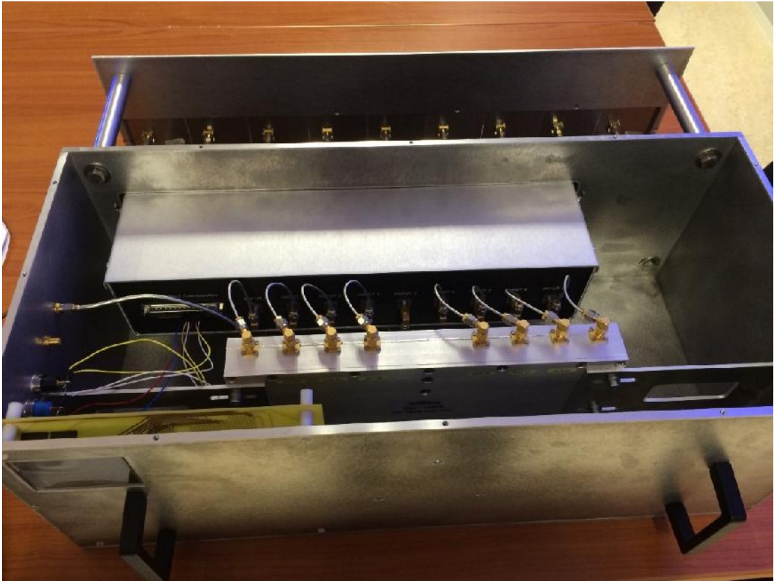
Figure IV-22: Prototype final réalisé du dispositif MARPEM complet.
