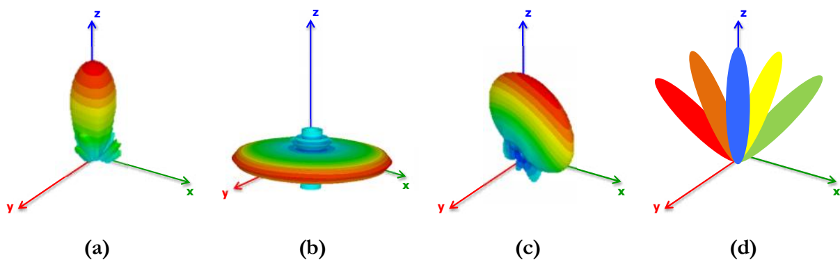
Figure II-1: Diagrammes de rayonnement (a) directives, (b) omnidirectionnels, (c) sectoriels et (d) agiles.
