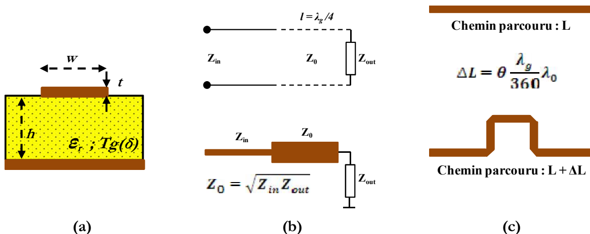
Figure 4: (a) Ligne microruban et ses paramètres (b) Transformateur d'impédance à ligne quart d'onde et (c) Ligne à retard de phase en technologie microruban.
