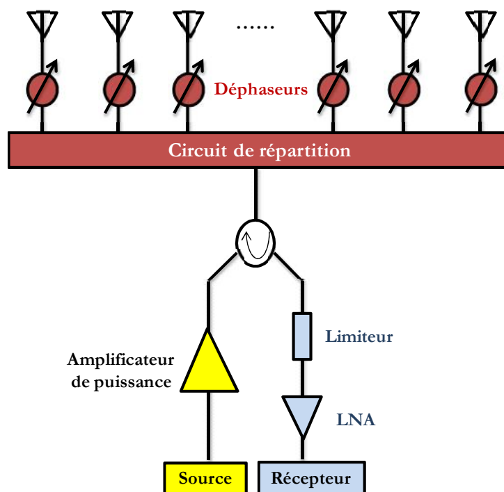
Figure I-1: Synoptique d'une architecture passive à balayage avec un déphaseur pour chaque élément rayonnant.
