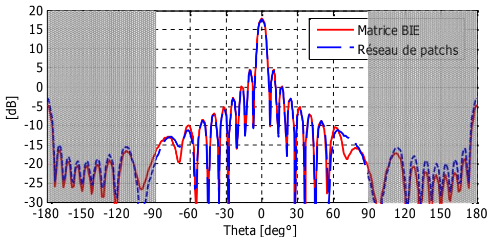
Figure II-24: Comparaison de diagrammes de rayonnement dans la direction axiale ( f_0 = 8 \text{ GHz} ).
