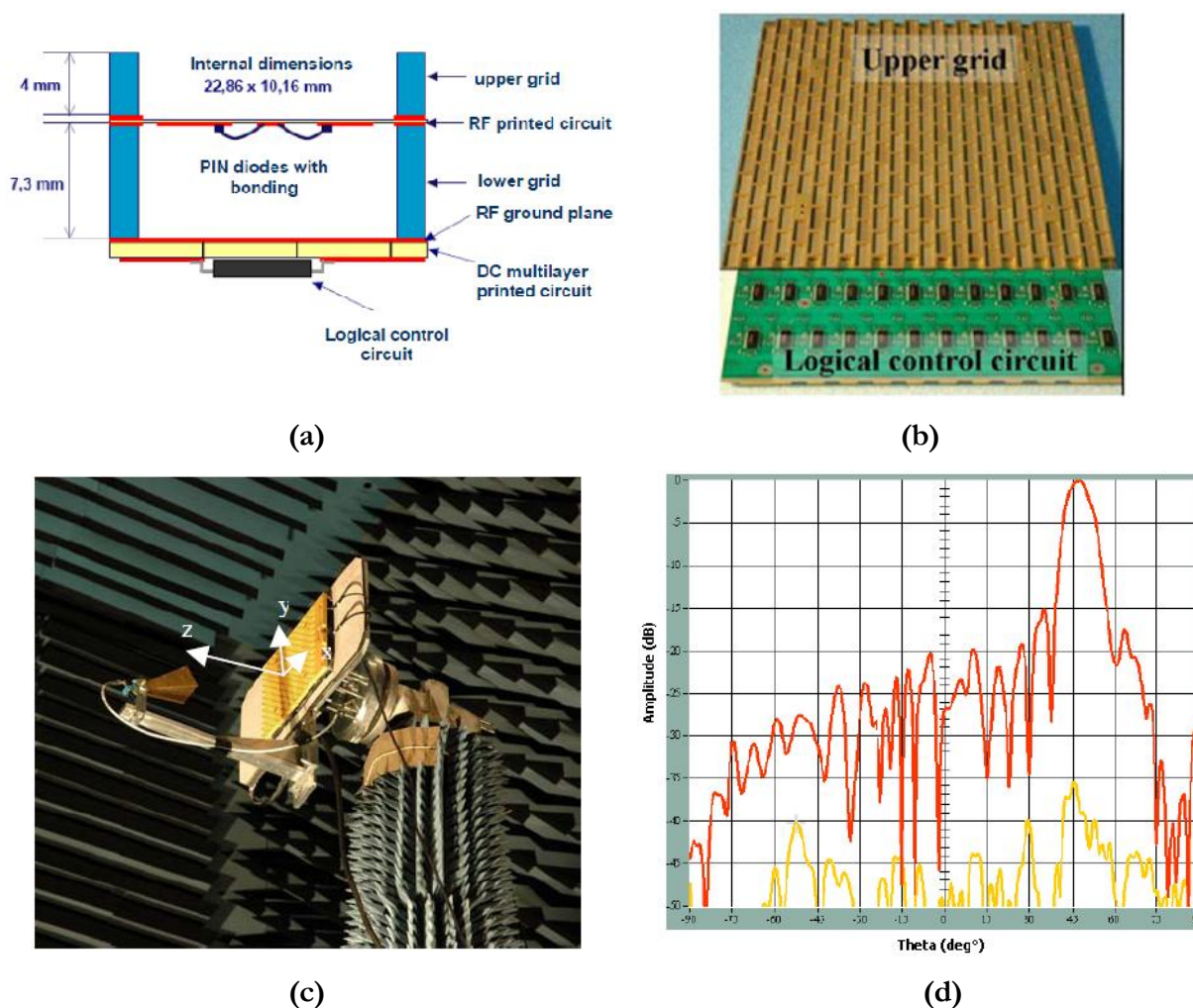
Figure 6: (a) Cellule (b) Le panneau en présence du circuit de contrôle (c) Antenne finale en chambre anhoïade du CNES et (d) Diagrammes mesurés ( \theta=45^\circ , \varphi=90^\circ ).
