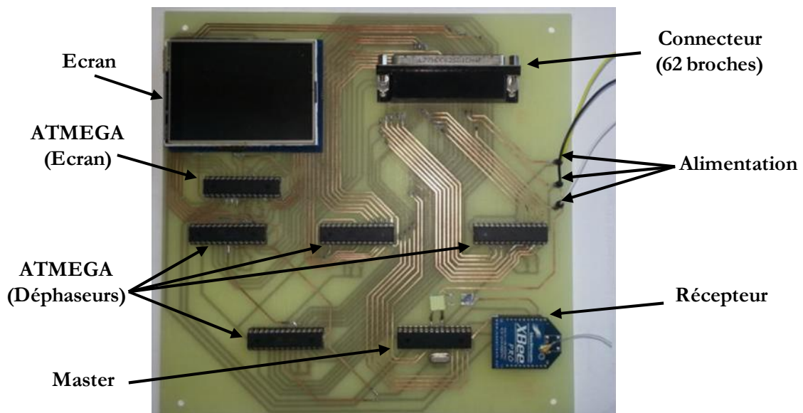
Figure IV-20: Carte de pilotage finale réalisée.
