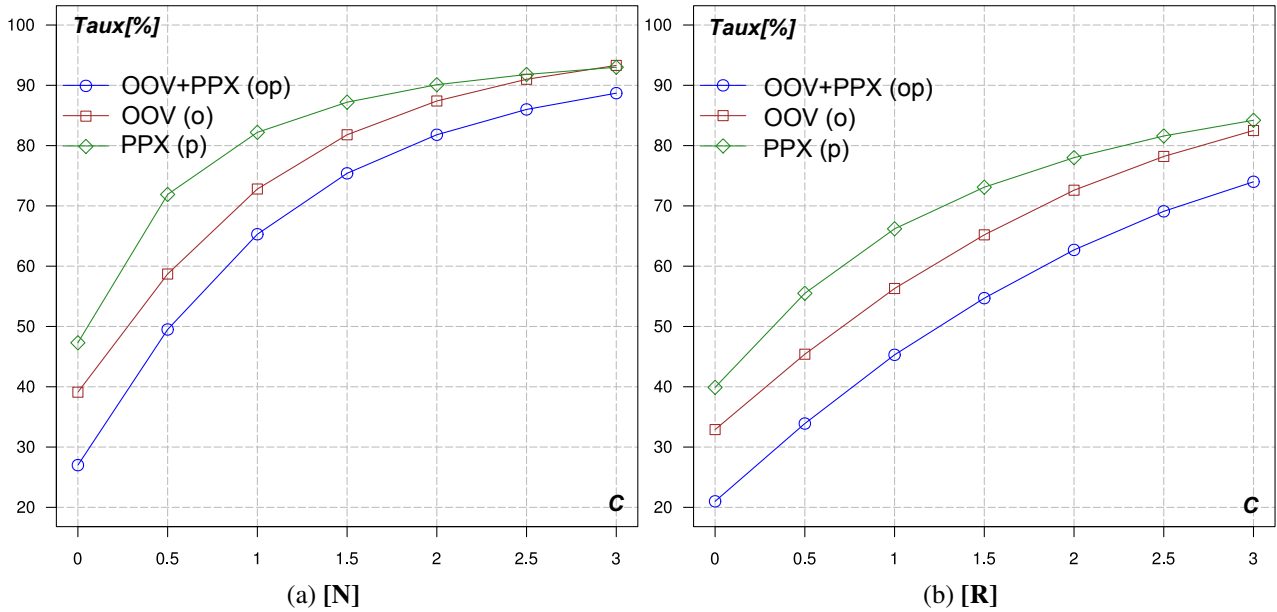
FIGURE 3.5 – Taux de sélection de documents (en pourcentage) à l'application de la méthode d'évaluation de la pertinence intrinsèque de documents sur le corpus d'évaluation Quaero Q07fr de 499 734 pages web. c : constante de sélection. oov, ppx et oov+ppx : fonction de sélection. N et R : méthode d'estimation normale en 3.5a versus restreinte en 3.5b des distributions OOV et PPX servant à établir les seuils de pertinence des fonctions de sélection.
