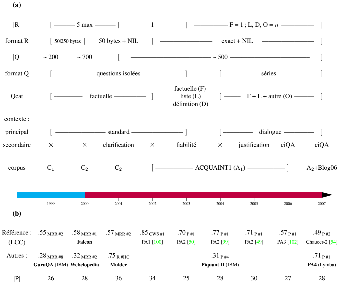
FIGURE 2.7 – Exemples de critères d'évaluation utilisés dans les campagnes QR (TREC 1999-2007). (a) Critères . |Q| et |R| : nombre total de questions et de réponses (distinctes) autorisées. format R : format de réponses autorisé ; en bytes (50 ou 250) ou en terme d'exactitude : correcte, incorrecte, etc. ou NIL (aucune réponse n'existe dans le corpus de travail). format Q : format de la question. contexte : challenges QR principal et secondaire (× : pas de challenge). Qcat : catégorie de question. corpus : corpus de travail. (b) Performances de systèmes QR sur les campagnes TREC 1999-2007 . Le format des performances systèmes fournies est : score M #rang . M : la mesure QR considérée pour l'année. MRR : moyenne des rangs réciproques, P : précision, R : rappel et CWS : Combined Weighted Score. #rang : position des participants dans le classement TREC de l'année (HC : hors compétition). Les résultats fournis de 1999 à 2001 ne concernent que les challenges avec réponses au format 50 bytes. Les résultats fournis de 2003 à 2007 ne concernent que les questions factuelles. En gras, les systèmes dont nous avons parlé dans le chapitre. PA : le système Power Answer du LCC (v1 à v3) puis de Lymba (v4). |P| : nombre de participants.
