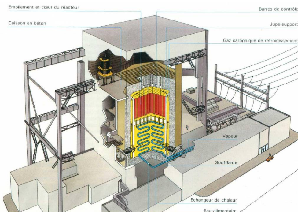
Figure 1 : Vue schématique d'un réacteur UNGG
