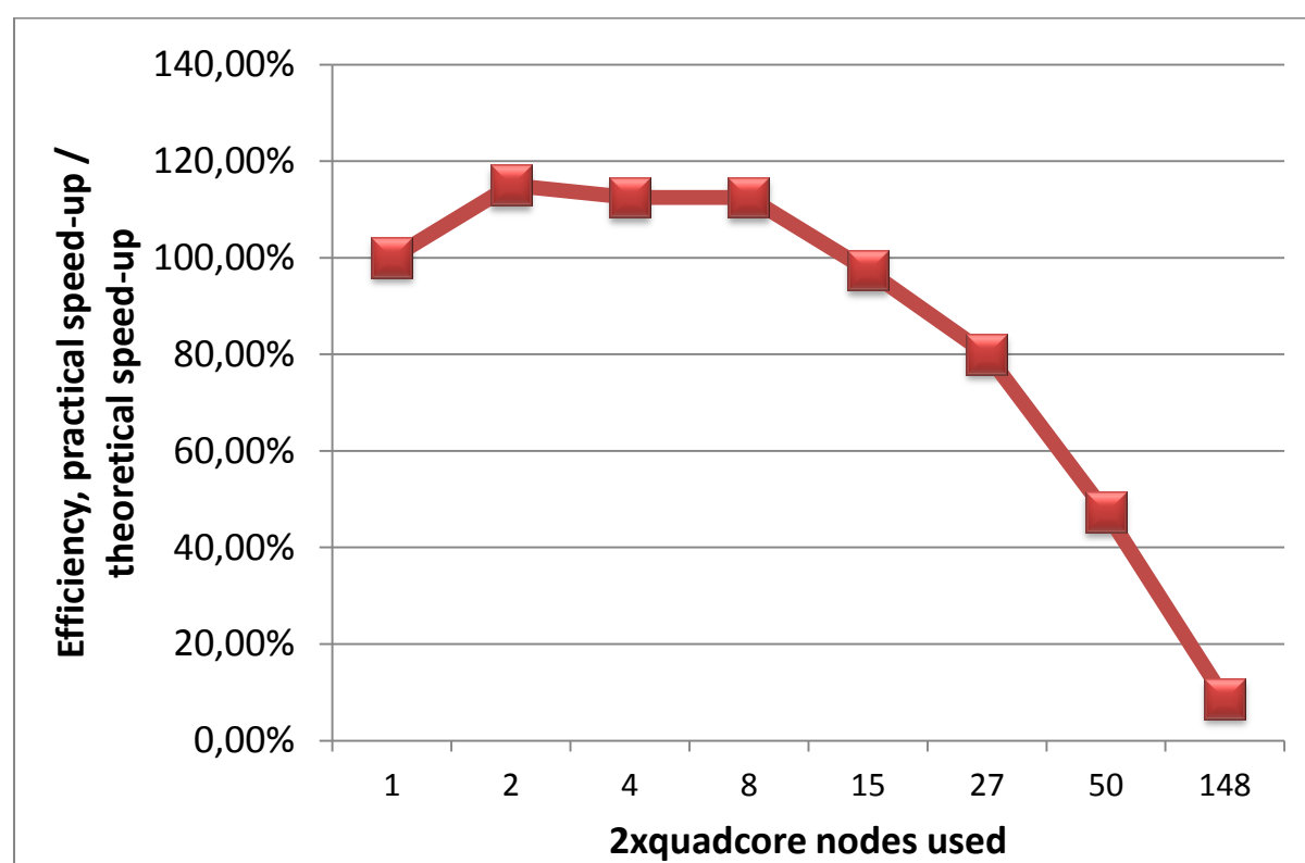
Figure 39. Efficacité d'ERAM sur la machine Titane.
