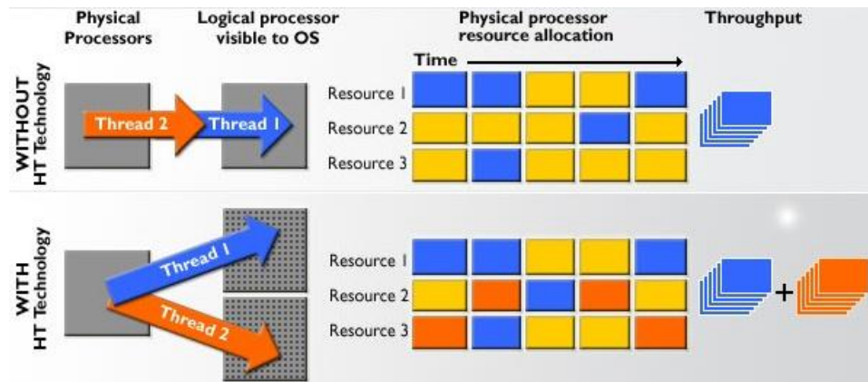
Figure 7. Fonctionnement de l'Hyperthreading sur processeur Intel.
