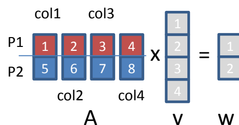
Figure 22. Produit matrice-vecteur par colonnes (axpy) avec deux processeurs P1 et P2. P1 traite son élément de la colonne 1, calculant w(1) = w(1) + \text{col1}(1) * v(1) . P2 fait de même : w(2) = w(2) + \text{col1}(2) * v(1) . Les deux processus passent ensuite à la colonne 2 et l'élément 2 du vecteur V pour effectuer les mêmes opérations, et continuent jusqu'au parcours de toutes les colonnes.
