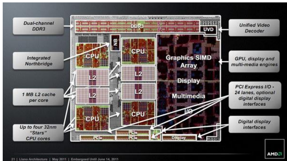
Figure 6. Surface d'un processeur AMD Fusion intégrant puce graphique et cœurs x86 standards.
