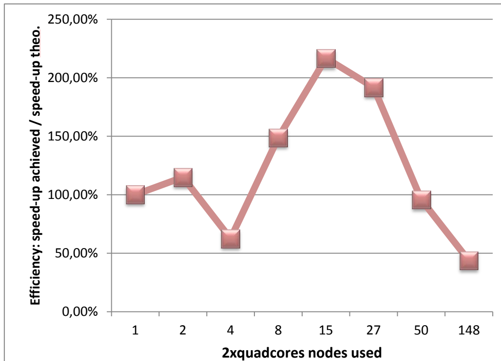
Figure 47. Efficacité de MERAM selon le nombre de nœuds de Titane utilisés.
