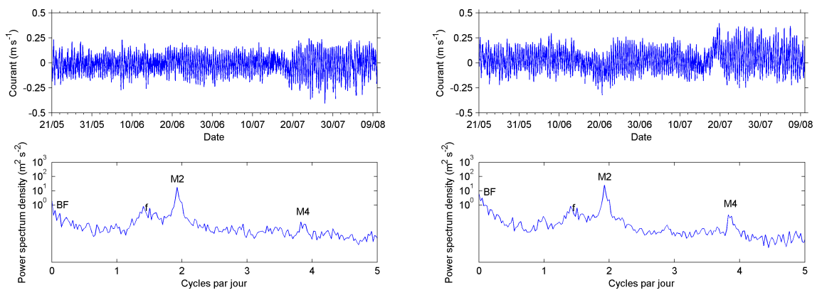
(c) Courant U au fond et sa TF
