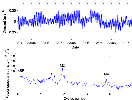
(d) Courant V au fond et sa TF
