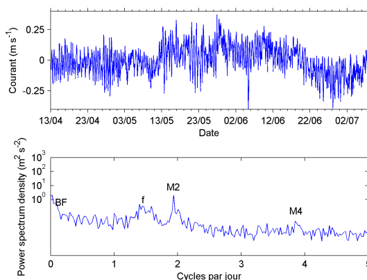
(b) Courant V en surface et sa TF
