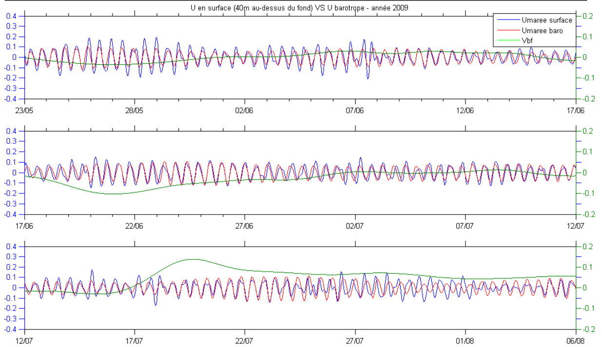
FIG. IV.9 – U en surface - Données ADCP 2009
