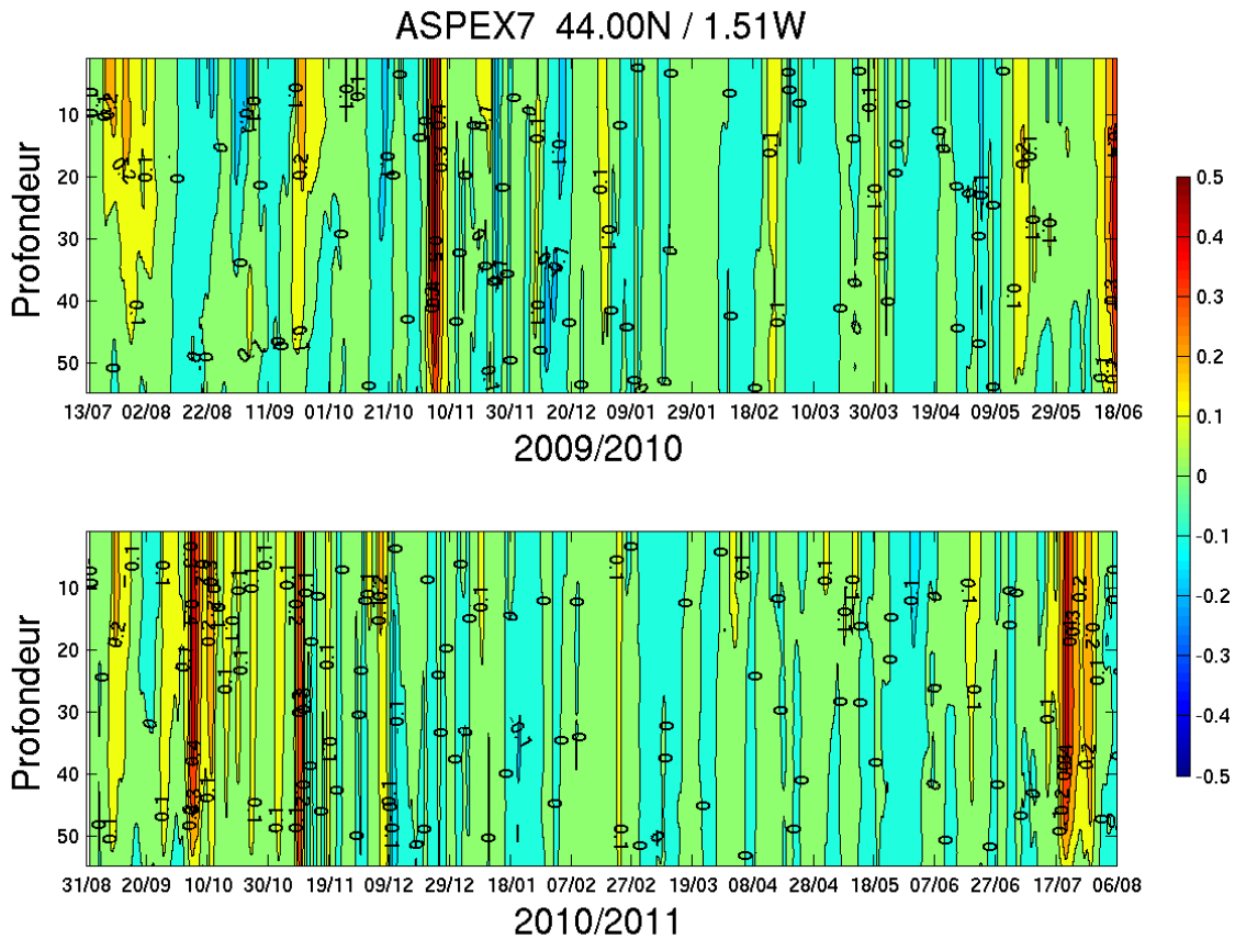
FIG. IV.29 – Courants longshore sur la radiale à 44°N sur l’isobathe 60m - données ASPEX
