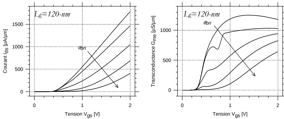
Fig. 2.51 : Courant de drain I_{ds} et transconductance G_{me} en fonction de la tension de grille V_{gs} pour différentes hauteurs de barrière aux électrons variant de 0 à 0.2 eV par pas de 0.05 eV. La tension de drain est fixée à 2 V.
