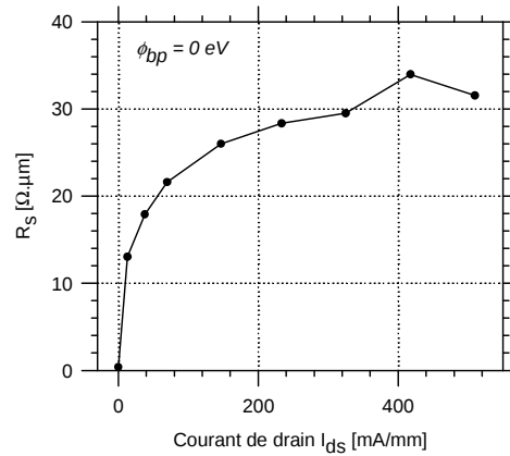
Fig. 3.55 : Résistance R_s extraite tracée en fonction du courant de drain I_{ds} pour une tension de drain V_{ds} = -2 V , pour une hauteurs de barrière de nulle et pour une distance de non-recouvrement nulle.
