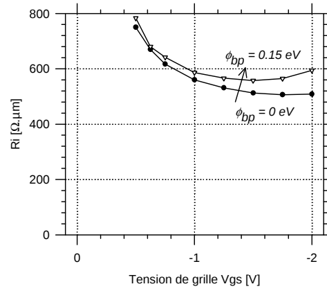
Fig. 3.53 : Résistance R_i extraite et tracée en fonction de la tension de grille V_{gs} pour une tension de drain fixée à -2 V et pour deux hauteurs de barrière. Rappelons que le terme de vitesse de recombinaison est fixé très grand.
