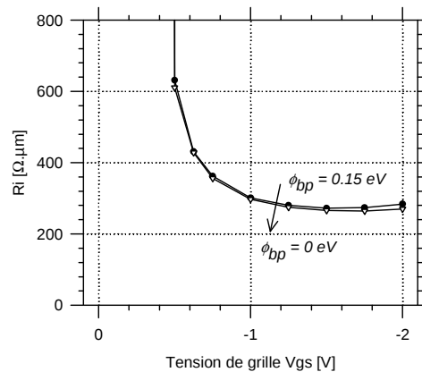
Fig. 3.54 : Résistance R_i tracée en fonction de la tension de grille V_{gs} pour une tension de drain fixée à -2 V et une hauteur de barrière nulle, calculée suivant l'expression R_i g_m \approx 0.5R avec R retenue à 0.2. Rappelons que le terme de vitesse de recombinaison est fixé très grand.
