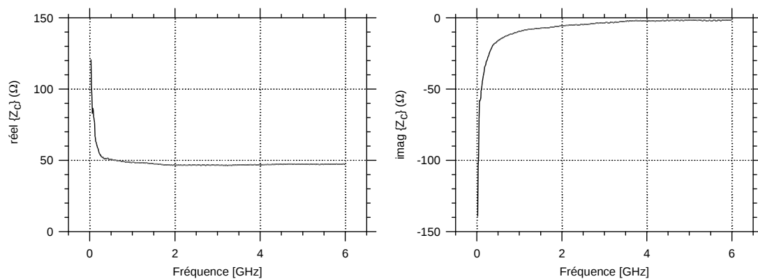
Fig. 3.12 : Impédance caractéristique complexe d'une ligne coplanaire de 300-μm mesurée sur le substrat faiblement résistif (SRS). L'expression pour extraire Z_c est rappelée à l'Annexe E.
