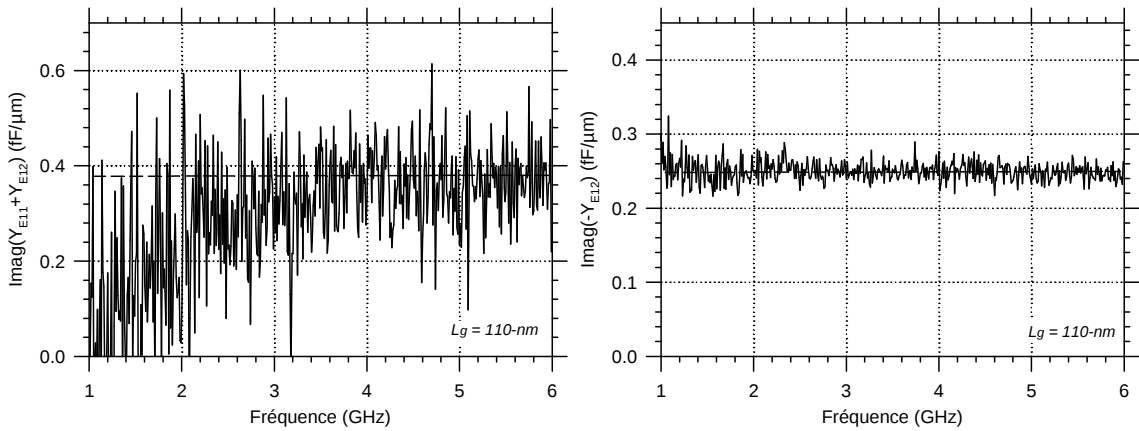
Fig. 3.20 : Extraction des capacités extrinsèques C_{gse} et C_{gde} à partir des parties imaginaires de (Y_{E11} + Y_{E12}) et (-Y_{E12}) . Les capacités sont estimées à 0.38 \text{ fF/}\mu\text{m} et 0.25 \text{ fF/}\mu\text{m} ( V_{ds} = V_{gs} = -1.5 \text{ V} ). Le ratio est \sim 5 .
