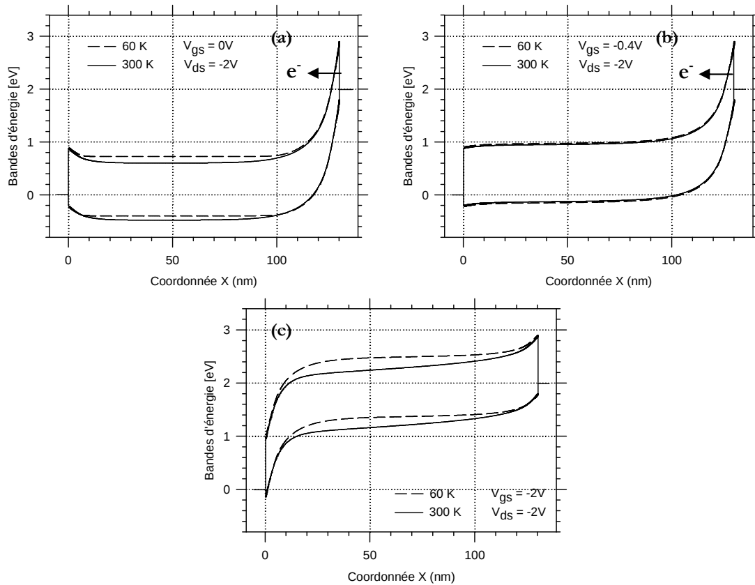
Fig. 2.35 : Bandes d'énergie tracées pour différentes tensions de grille, V_{gs} = 0\text{ V} (a), V_{gs} = -0.4\text{ V} (b) et V_{gs} = -2\text{ V} (c) et pour deux températures, 300 K et 60 K. Les différents régimes correspondent aux points reportés sur le diagramme d'Arrhenius à la Fig. 2.34.
