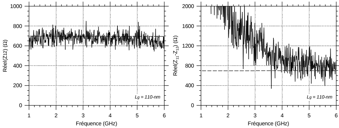
Fig. 3.23 : Extraction des résistances séries R_s (à gauche) et R_g (à droite) à partir des parties réelles de (Z_{12}) et (Z_{11}-Z_{12}) . R_s et R_g sont approximées à \sim 700 \, \Omega ( V_{ds} = V_{gs} = -1.5 \, V ).
