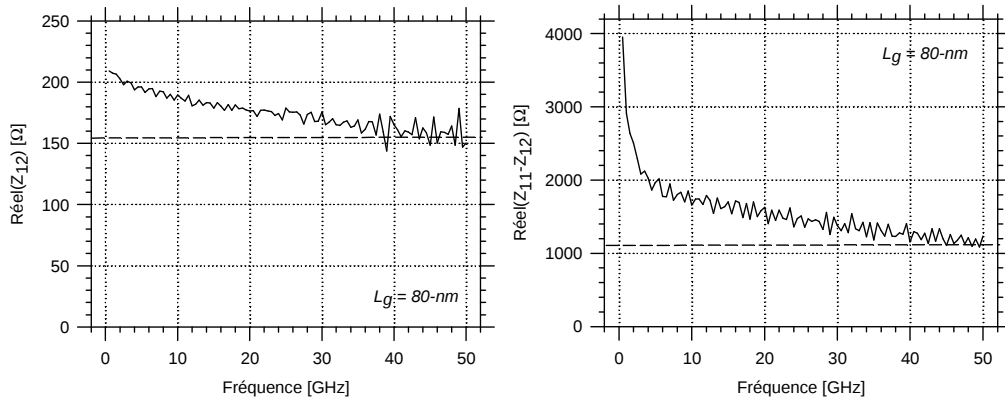
Fig. 3.43 : Parties réelles des paramètres Z_{12} et (Z_{11}-Z_{12}) à V_{sg} = 1.2 V et V_{dg} = -0.8 V (équivalent à V_{ds} = -2 V et V_{gs} = -1.2 V).
