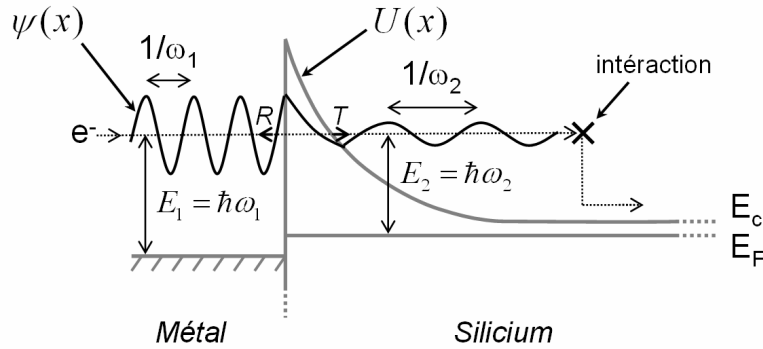
Fig. 1.31 : Traduction schématique de l'équation de Schrödinger appliquée à une barrière Schottky polarisée. \Psi(x) représente l'amplitude de probabilité de présence de l'électron émis à une énergie E_1 dans le métal (considérer ici comme structuré, comme c'est le cas du siliciure de platine) et positionné à une énergie E_2 dans le semi-conducteur. R et T représentent respectivement la réflexion de l'onde électronique sur la barrière et la transmission à travers la barrière. Dans la barrière, \Psi(x) décroît exponentiellement. Dans cette schématique, les énergies E_1 et E_2 se distinguent à cause de la différence de potentiel, ce qui amène l'électron à observer deux vitesses électroniques distinctes (De Broglie).
