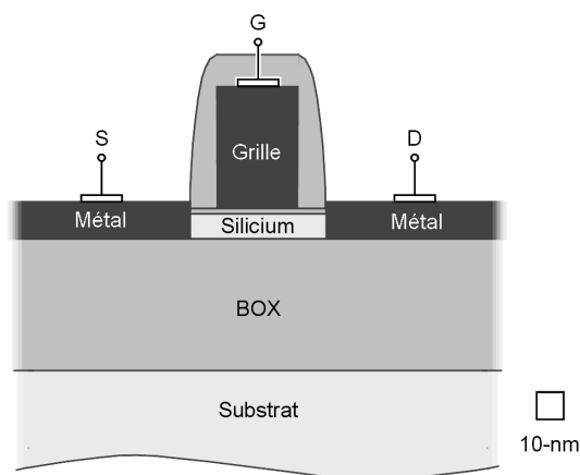
Fig. 1.1 : Schématique d'un transistor SB-MOSFET sur film SOI ultra fin fabriqué à l'IEMN dans le cadre du projet METAMOS [1]. Les longueurs et des largeurs sont normalisées suivant un carré de longueur de coté équivalente à 10-nm. La longueur de grille est équivalente à 30-nm, l'épaisseur de silicium à 10-nm, l'épaisseur d'oxyde à 2-nm.
