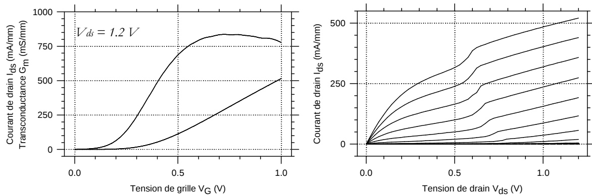
Fig. H.1 : Caractéristiques de courant et transconductance normalisées en fonction des tensions de grilles et de drain. La tension de grille variant de 0 à 1 V par pas de 0.1 V. Notons que la prise substrat est laissée flottante, ce qui amène à un effet kink que l'on peut observer sur la caractéristique I_{ds}-V_{ds} .
