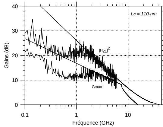
Fig. 3.27 : Comparaison entre les gains mesurés et simulés en fonction de la fréquence ( V_{ds} = V_{gs} = -1.5\text{ V} ).
