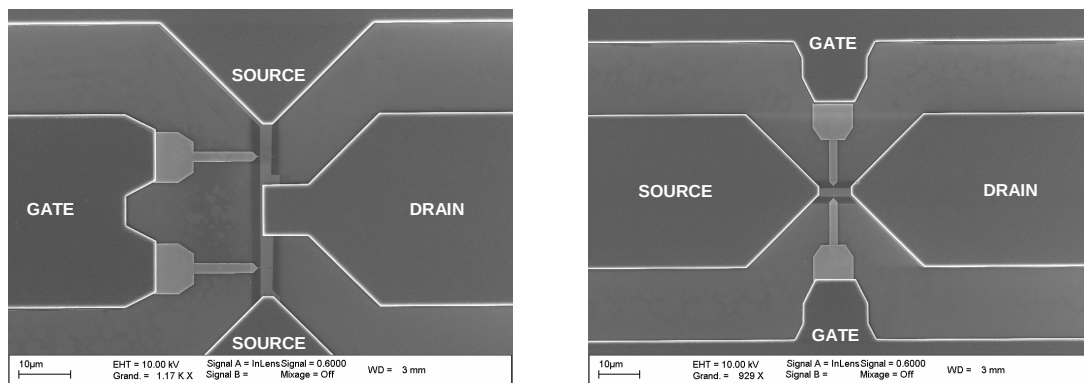
Fig. 3.33 : Vue au microscope électronique des topologies de transistors SB MOSFET configurées en source commune (à gauche) et grille commune (à droite). Les doigts de grille sont tournés de 90° entre ces deux structures. A noter que grâce aux deux accès de grille, la topologie grille commune est équivalente à une topologie source commune avec deux doigts de grille dont la largeur des doigts est égale à une demi largeur de doigt de grille.
