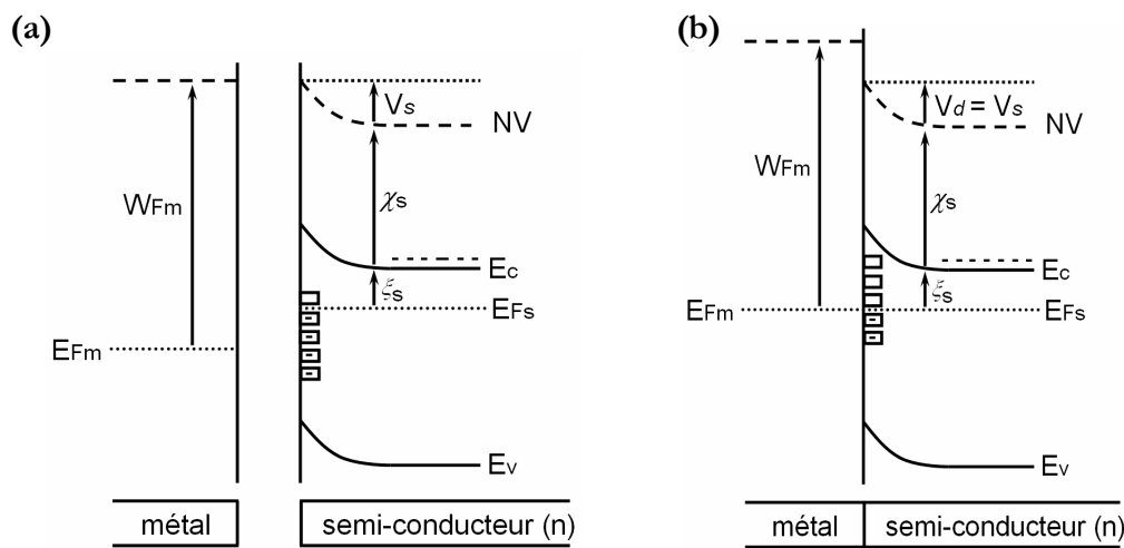
Fig. 1.27 : Schématisation des courbures de bandes lorsque un semi-conducteur de type n comporte des états d'interface. Dans ce cas présent, les pièges sont de type accepteurs d'électrons. Puisque les électrons sont tentés de quitter la bande de conduction, il se forme une zone de charge d'espace qui a pour effet de faire apparaître une barrière de potentiel (a). Lorsque les deux matériaux sont mis en contact (b), les niveaux de Fermi doivent s'aligner. Les électrons aux états d'énergies les plus proches du niveau de Fermi sont privilégiés pour être transféré dans le métal et ce sans modifier les courbures des bandes. Ainsi, la barrière de potentiel reste conditionnée par les états d'interface sans être affectée par le travail de sortie du métal.
