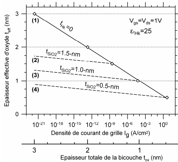
Fig. 1.16 : Epaisseur d'oxyde en fonction de la densité de courant de grille I_g (ligne continue) (1). (1) est la référence car l'épaisseur n'est constituée que de SiO 2 et dans ce cas, l'épaisseur t_{ox} est égale à t_{eff} . Les points sont issus de la Fig. 1.14 lorsque V_{ds} = V_{gs} = 1\text{ V} . Superposée l'épaisseur effective d'oxyde extrapolée en fonction de l'épaisseur totale d'oxyde et donc du courant de grille pour différentes épaisseurs d'oxyde de silicium SiO 2 variant de 0.5 (2), 1 (3) à 1.5-nm (4) (ligne pointillée). La bicouche est constituée d'un matériau SiO 2 et un matériau High- \kappa dont la permittivité relative est égale à 25, correspondant typiquement à celle de l'oxyde d'hafnium (HfO 2 ). On considère ici que les « masses effectives » dans les oxydes sont identiques [17].
