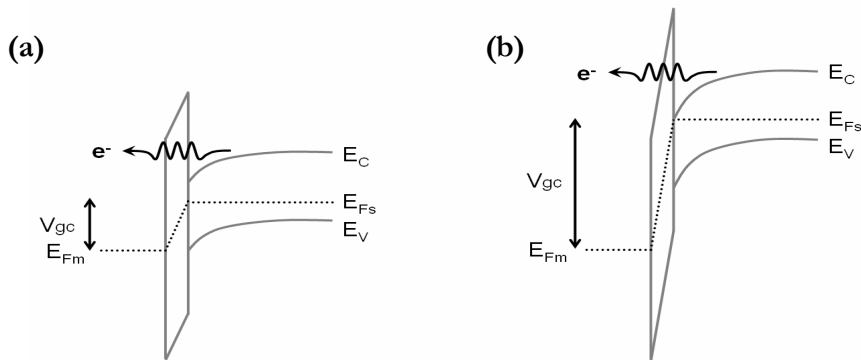
Fig. 1.15 : Schématisation des courbures de bandes et de l'effet tunnel, majoritairement causé par effet tunnel direct (champ électrique faible) (a) et par effet Fowler-Nordheim (champ électrique élevé) (b). V_{gc} est la tension grille-à-canal.
