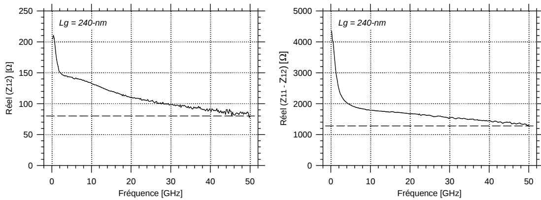
Fig. 3.36 : Parties réelles non-normalisées de R_{\text{réel}}(Z_{12}) et R_{\text{réel}}(Z_{11}-Z_{12}) en fonction de la fréquence à V_{ds} = -2 V , V_{gs} = -1.5 V . R_s et R_g sont extraites approximativement à 80 \Omega et 1150 \Omega .
