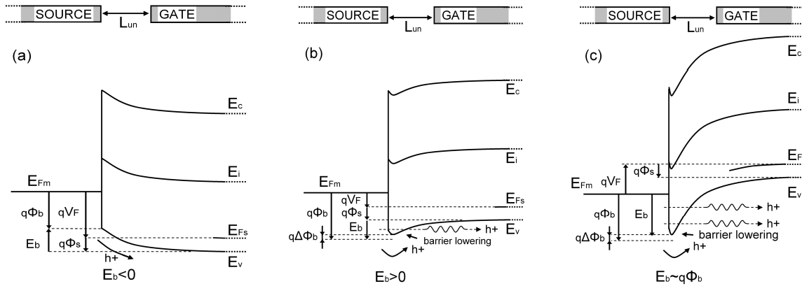
Fig. 1.22 : Schématisation des courbures de bandes d'énergies à l'interface Schottky côté source à V_{gs} = 0\text{ V} (a), moyenne et forte polarisation négative de grille (b, c) (cas d'un SB MOSFET type p ). La hauteur de barrière \Phi_b est choisie importante dans le but d'observer la déformation des bandes d'énergies. L'émission thermoïonique (TE), l'émission tunnel (FE) et l'émission thermoïonique par effet de champ (TFE) sont présentées. L'abaissement de barrière \Delta\Phi_b induit par l'effet de la charge image est également schématisé (b, c).
