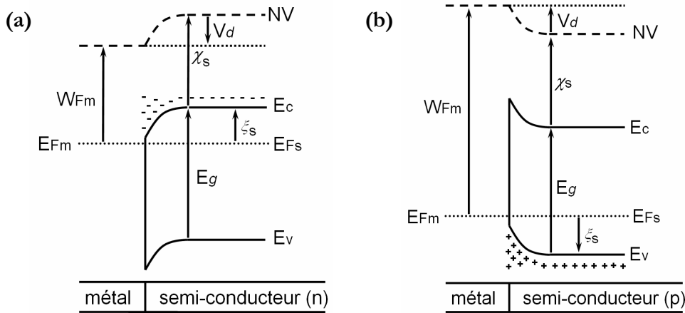
Fig. 1.24 : Diagrammes d'énergie lorsque le contact est Ohmique dans les cas d'un semi-conducteur dopé de type n (a) et p (b). Ainsi le transport est majoritairement mue par les électrons (a) et les trous (b) respectivement.
