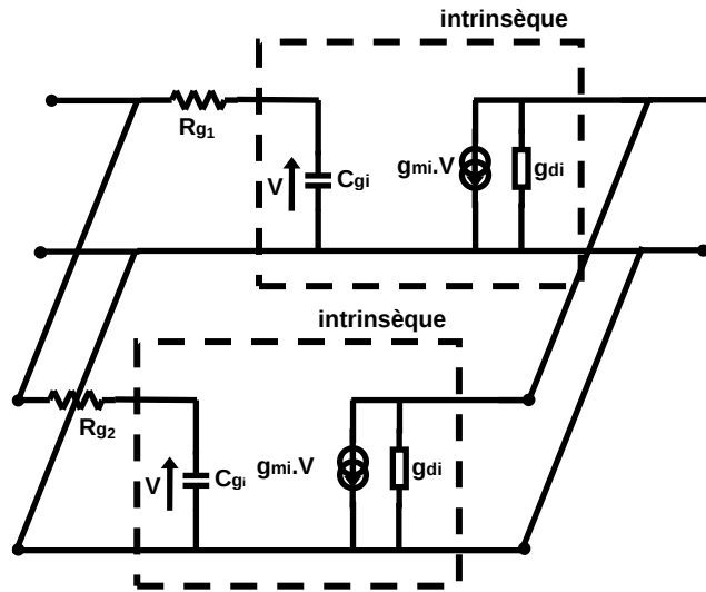
Fig. 3.49 : Schéma équivalent petit signal simplifié de deux doigts d'un transistor MOSFET.
