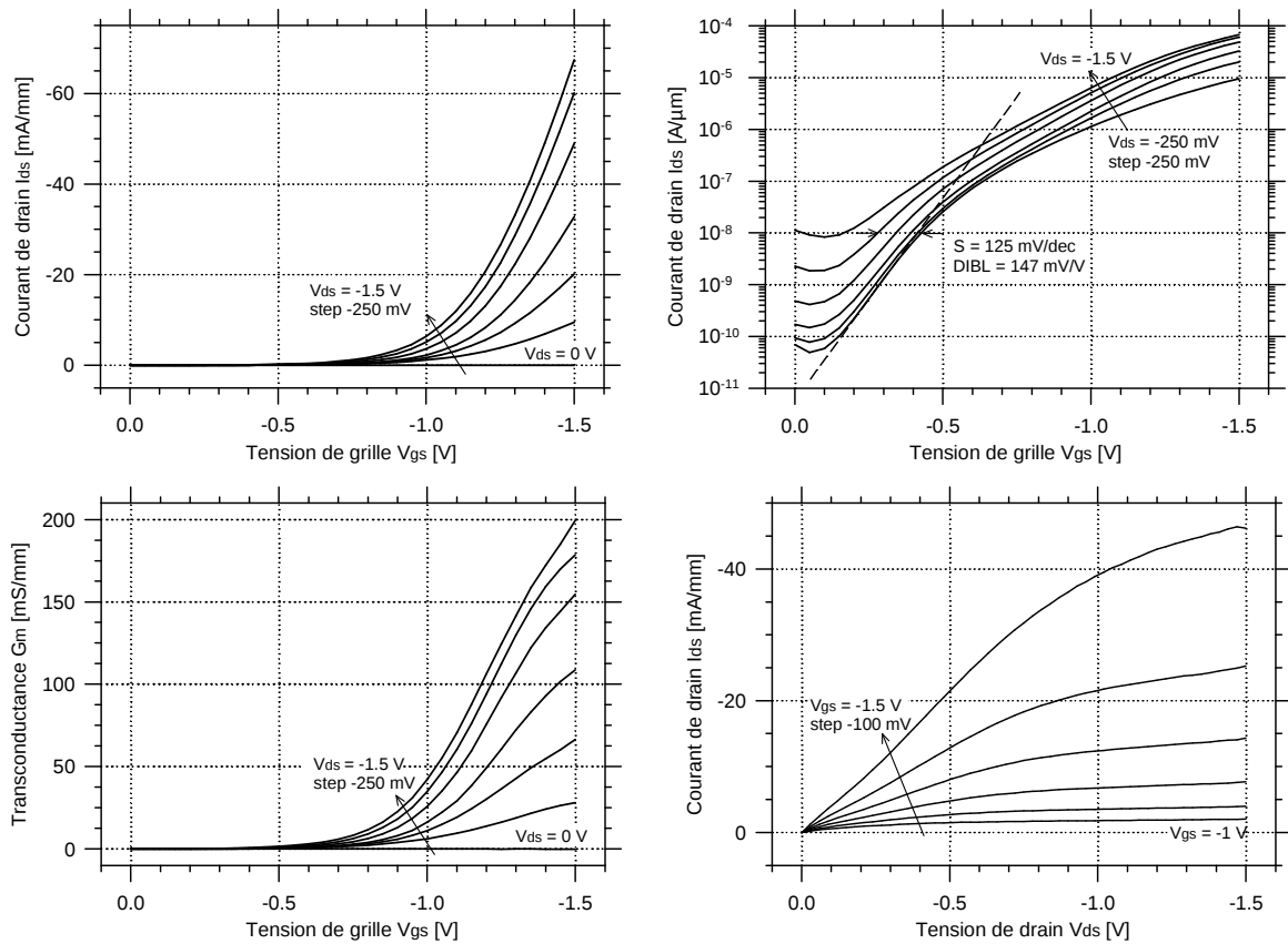
Fig. 3.15 : Caractéristiques statiques normalisées I_{ds}\text{-}V_{gs} (a), \log(I_{ds})\text{-}V_{gs} (b), G_m\text{-}V_{gs} (c), I_{ds}\text{-}V_{ds} (d). Ce composant présente un courant I_{on} de 80\text{ }\mu\text{A}/\mu\text{m} , une transconductance maximum de 200\text{ }\mu\text{S}/\mu\text{m} à V_{ds} = V_{gs} = -1.5\text{ V} .
