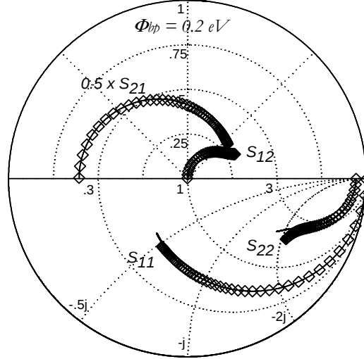
Fig. 3.60 : Comparaison entre le modèle non quasi-statique rétro-simulé et les paramètres S issus du transistor SB MOSFET pour V_{ds} = -2 V, V_{gs} = -2 V. Les symboles correspondent aux points issus du simulateur de composant et les lignes du modèle SSEC non quasi-statique. La fréquence varie de 100 MHz à 100 GHz. La hauteur de barrière est définie à 0.2 eV.
