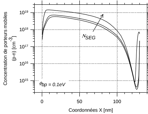
Fig. 2.49 : Concentration de porteurs mobiles ( p-n ) le long du canal pour différentes concentrations N_{SEG} variant de 10^{12} , 5 \times 10^{18} à 10^{20} \text{cm}^{-3} . La longueur de grille est de 120-nm, les largeurs de recouvrement de 5-nm. L'abscisse zéro correspond à l'interface du contact Schottky de source. La largeur du film de ségrégation est fixée à 5-nm. Le point de polarisation est considéré à V_{ds} = -2 V et V_{gs} = -1 V.
