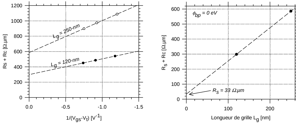
Fig. 3.56 : Extraction de la résistance R_s par la méthode à froid à partir des paramètres AC provenant des simulations.
