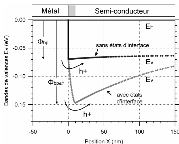
Fig. 1.29 : Simulation des courbures de bandes de valence pour un contact Schottky avec et sans états d'interface. La densité d'états d'interface de type donneur est de 10^{12} \text{ cm}^{-2} . Le niveau d'énergie des états d'interface est situé à 0.3 eV sous la bande de conduction. La concentration de dopants dans le silicium est de 2 \times 10^{15} \text{ cm}^{-3} et la diode est placée à la température de 100 K. Nous observons que si la hauteur de barrière est de 70 meV dans le cas d'une diode Schottky idéale, la barrière effective dans le cas d'une diode comprenant des états d'interface augmente à près de 150 meV.
