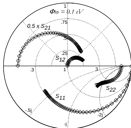
Fig. 3.59 : Comparaison entre le modèle non quasi-statique rétro-simulé et les paramètres S issus du transistor SB MOSFET pour V_{ds} = -2\text{ V} , V_{gs} = -2\text{ V} . Les symboles correspondent aux points issus du simulateur de composant et les lignes du modèle SSEC non quasi-statique. La fréquence varie de 100 MHz à 100 GHz. La hauteur de barrière est définie à 0.1 eV.
