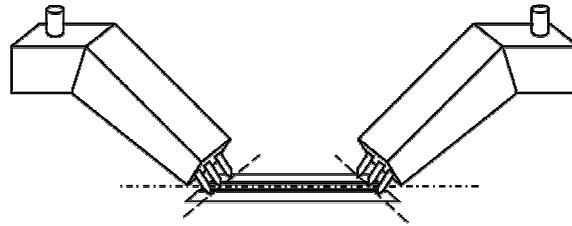
Fig. 3.4 : Schématic des pointes RF posées sur un motif correspondant à une ligne associée aux plans de référence définies aux bords des pointes après l'étalonnage.
