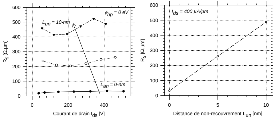
Fig. 3.57 : Résistance R_s extraite tracée en fonction du courant de drain I_{ds} pour une tensions de drain V_{ds} = -2V , pour une hauteur de barrière de nulle et pour différentes largeurs d'underlap variant de 0, 5 à 10-nm.
