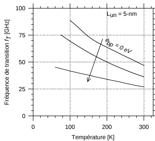
Fig. 2.33 : Fréquence de coupure en courant en fonction de la température à la polarisation V_{gs} = V_{ds} = -2 V. Les hauteurs de barrière sont définies à 0, 0.1 et 0.2 eV. La largeur de non-recouvrement L_{un} est fixée à 5-nm
