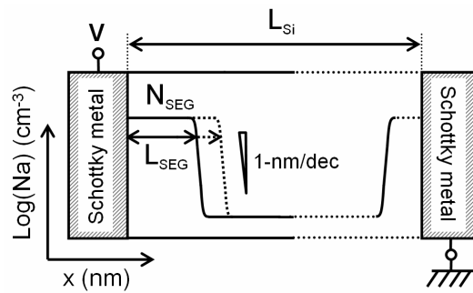
Fig. 2.41 : Schématique de diodes en vis-à-vis dont les contacts sont ségrégés.
