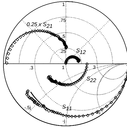
Fig. H.4 : Comparaison entre le modèle non quasi-statique rétro-simulé et les paramètres S issus du transistor à V_{ds} = 1.2\text{ V} , V_{gs} = 0.7\text{ V} . Les symboles correspondent aux points issus des mesures et les lignes du modèle SSEC non quasi-statique. La fréquence varie de 500 MHz à 100.5 GHz par pas de 2 GHz.
