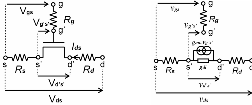
Fig. 1.17 : Schémas électriques en statique grand signal (a) et petit signal (b) d'un transistor MOSFET conventionnel avec la prise en compte des résistances de source R_s et drain R_d ainsi que de grille R_g .
