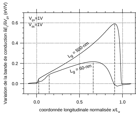
Fig. 1.10 : Dynamique d'amplitude de la bande de conduction avec la tension de grille \delta E_c / \delta V_{gs} le long du canal au point de polarisation V_{gs} = V_{ds} = 1\text{ V} pour deux longueurs de grille 60-nm et 500-nm.
