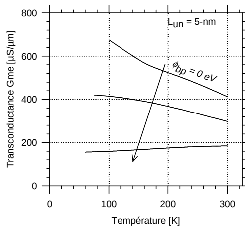
Fig. 2.32 : Transconductance G_{me} en fonction de la température pour différentes hauteurs de barrière variant de 0, 0.1 à 0.2 eV. La largeur de non-recouvrement L_{un} est fixée à 5-nm.
