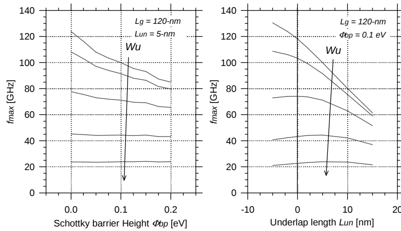
Fig. 2.30 : Extraction de la fréquence maximum d'oscillation f_{max} en fonction de la barrière Schottky (à gauche, L_{un}=5 -nm) et en fonction de la longueur de non-recouvrement (à droite, \phi_{bp} = 0.1 eV) pour différentes largeurs de doigt de grille W_u variant de 1, 2, 4, 8 to 16- \mu\text{m} ( R_{\square} = 10 \Omega/\square , V_{ds} = V_{gs} = -2 V).
