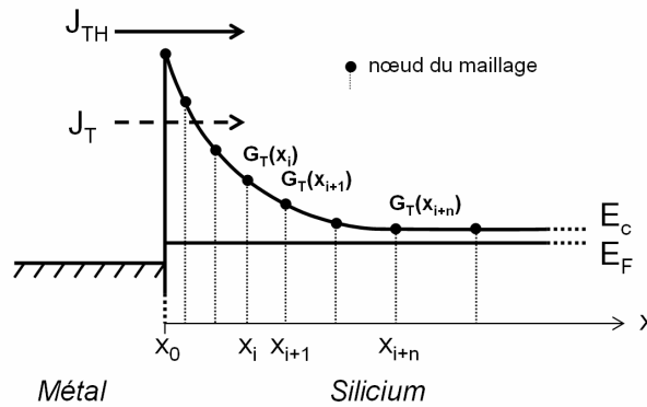
Fig. 2.3 : Représentation schématique du taux de génération de courant tunnel localisée implémentée dans un simulateur pour une barrière Schottky. J_{TH} et J_T sont respectivement les courants thermoionique et tunnel.
