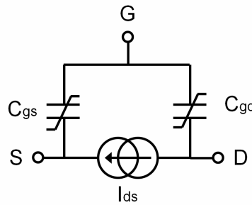
Fig. 1.5 : Représentation électrique idéale du transistor MOSFET.
