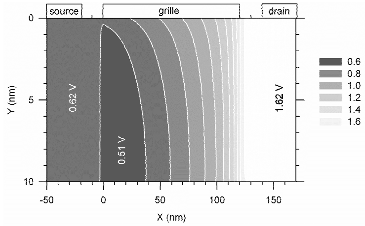
Fig. 1.8 : Lignes iso-potentiels pour une structure totalement désertée. Les lignes ne sont représentées uniquement que dans le silicium actif. La longueur de grille vaut 120-nm, l'épaisseur de silicium vaut t_{Si} = 10 -nm et l'épaisseur d'oxyde t_{ox} = 3 -nm. Les potentiels de grille et drain sont placés à 1 V.
