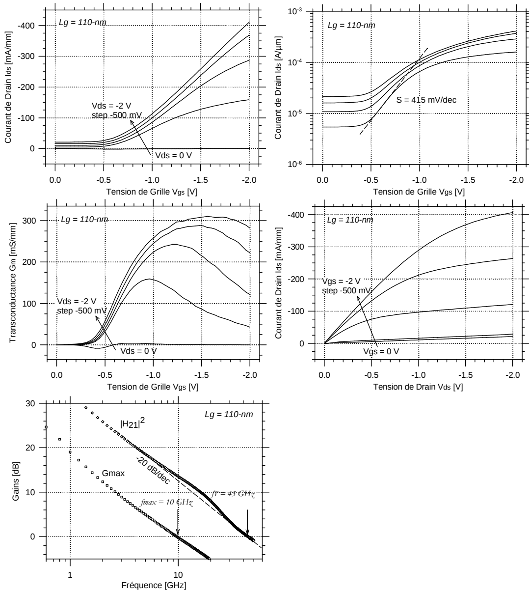
Fig. 3.31 : Caractéristiques statiques normalisées I_{ds} - V_{gs} (a), \log(I_{ds}) - V_{gs} (b), G_m - V_{gs} (c), I_{ds} - V_{ds} (d) et les figures de mérites AC des gains en courant |H_{21}|^2 et maximum G_{max} (e) pour un transistor de longueur de grille de 110-nm. Ce composant présente des fréquences f_T/f_{max} égale à 45/10 GHz à V_{ds} = -2.5 V et V_{gs} = -2 V.
