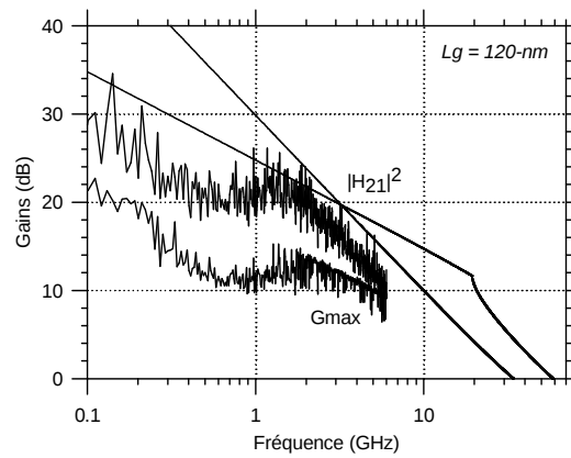
Fig. 3.29 : Comparaison entre les gains mesurés et simulés en fonction de la fréquence. Les gains simulés sont calculés en considérant R_g et R_s réduits d'un facteur 10.
