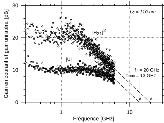
Fig. 3.17 : Gain en courant |H_{21}|^2 et gain unilatéral |U| pour un transistor de longueur de grille de 110-nm. Ce composant présente à V_{ds} = V_{gs} = -1.5\text{ V} un f_T de 20 GHz et un f_{max} de 13 GHz.
