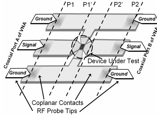
Fig. 3.7 : Schématisation d'une structures RF comprenant les accès coplanaires RF.
