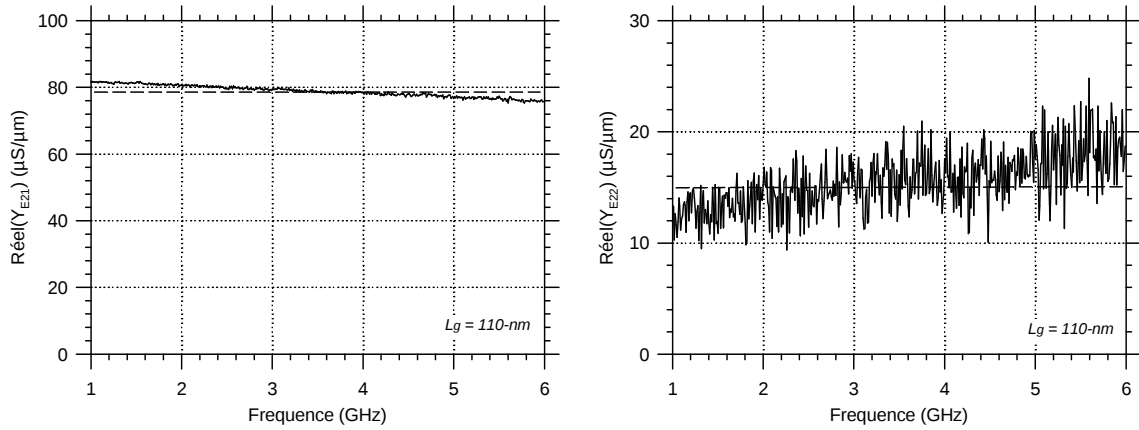
Fig. 3.19 : Extraction de la transconductance extrinsèque G_{me} (à gauche) et de la conductance de sortie G_{de} (à droite) à partir de la partie réelle de (Y_{E21}) et (Y_{E22}) respectivement. Les valeurs sont évaluées à environ 79 \text{ mS/mm} et 15 \text{ mS/mm} pour le transistor de longueur de grille de 110-nm. ( W_{tot} = 12\text{-}\mu\text{m} ) ( V_{ds} = V_{gs} = -1.5 \text{ V} ). Le ratio est \sim 5.5 .
