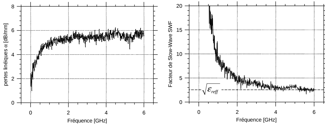
Fig. 3.13 : Constante d'atténuation normalisée (à gauche) et facteur de Slow-Wave (à droite) d'une ligne coplanaire de 300-μm mesurée sur le substrat faiblement résistif (SRS).
