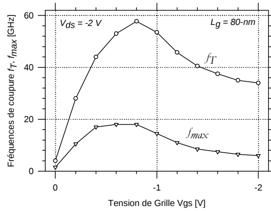
Fig. 3.40 : Extraction des fréquences de coupure f_T et f_{max} mesurée du transistor. La tension de drain est fixée à -2 V.
