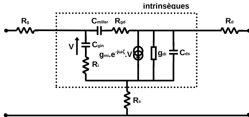
Fig. F.1 : Schéma équivalent petit signal non quasi-statique du transistor SOI MOSFET en saturation 1 . Les capacités C_{gin} et C_{miller} prennent compte implicitement les composantes de capacités parasites de recouvrement et de bord.
