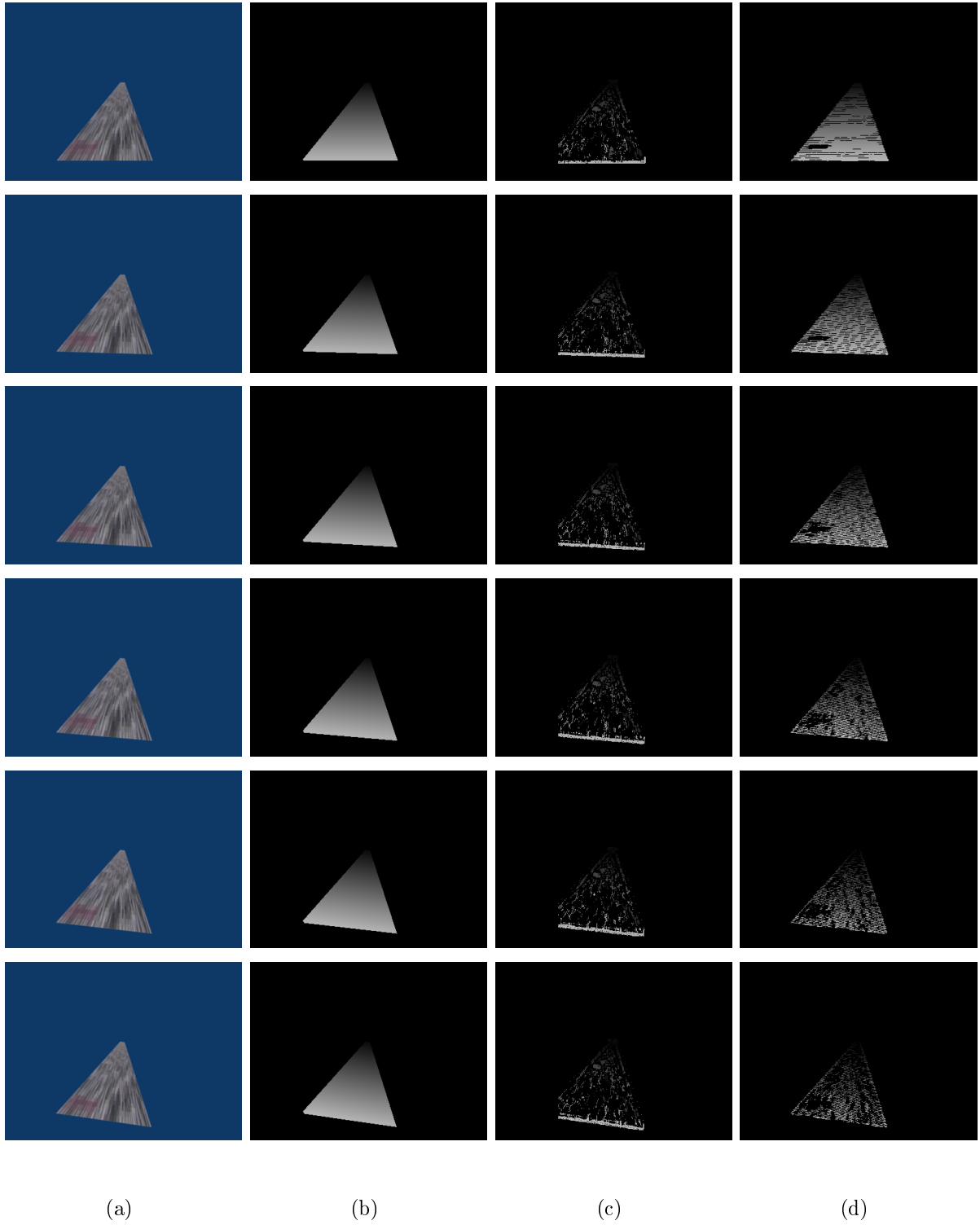
FIG. 3.18 : (a) Image droite, (b) Vérité-terrain, (c) Carte des disparités calculée par la méthode de Hirschmüller avec une fenêtre de taille 7 \times 9 et (d) Carte des disparités calculée avec notre méthode 1D (avec T_{dec} = 1 ).
