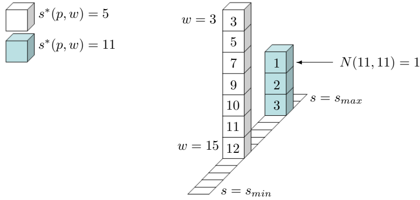
FIG. 3.7 : Volume réduit suivant la relation (3.7).
