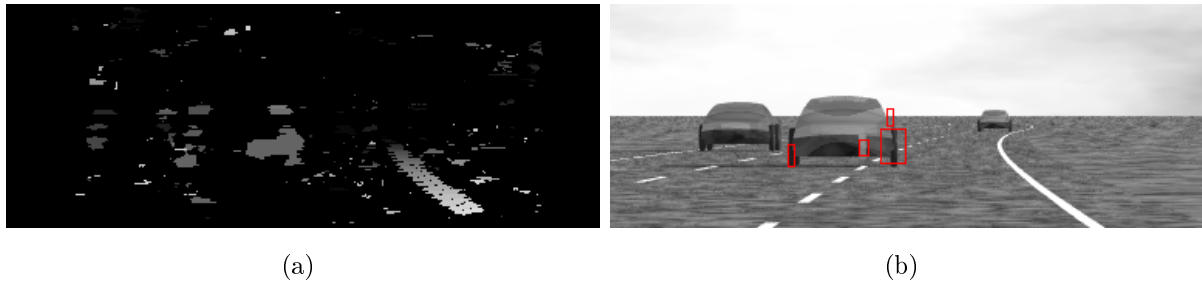
FIG. 4.21 : (a) Carte des disparités obtenues avec notre méthode 1D avec T_{dec} = 0.7 et une hauteur de fenêtre de 5 pixels, (b) Boîtes englobantes obtenues sur la carte des disparités (a) (ici, la caméra droite est sur-élevée de 5 cm).
