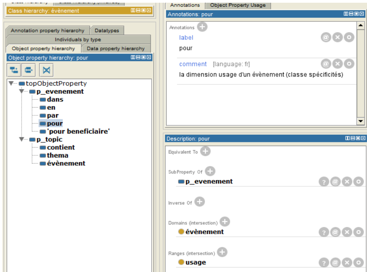
Figure 113 : Propriétés de l'ontologie Antimoine (essai D)
