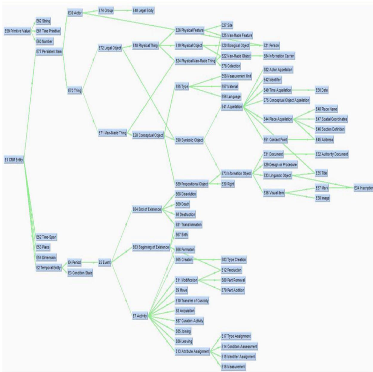
Figure 97 : Schéma général du CIDOC-CRM
