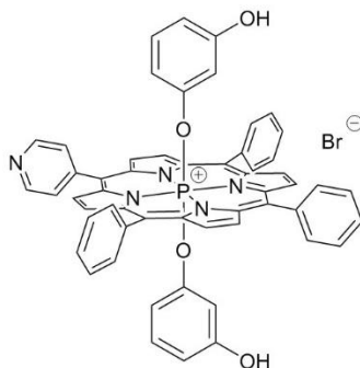
27, [P(MPyP)(OPhOH) 2 ] + Br -
