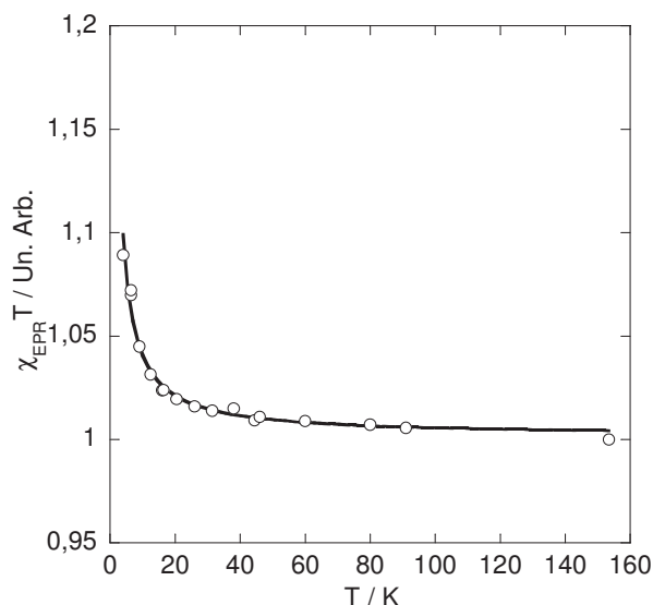
Figure 16 : Produit de la susceptibilité par la température en fonction de la température de la grille de Pym-Ph à 10^{-4} M dans l'acétonitrile.
