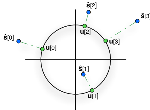
FIGURE 6.2 Construction du spectre \mathbf{u} du projeté P_B(\mathbf{s})
