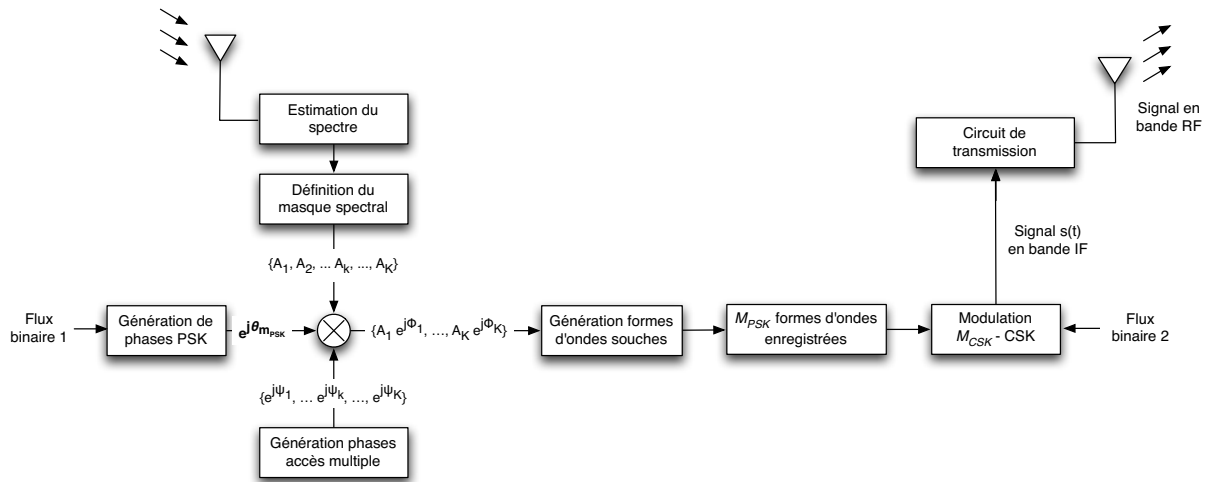
FIGURE 4.6 Modèle d'émetteur TDCS à modulation à flux CSK et PSK disjoints [Budi 08c]
