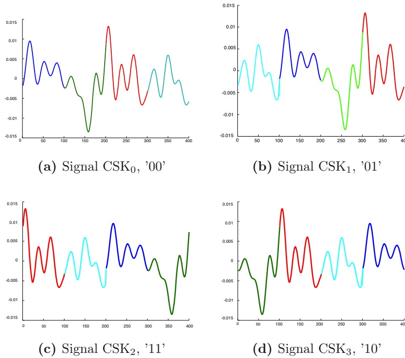
FIGURE 3.3 Exemple de signaux générés par la modulation CSK
