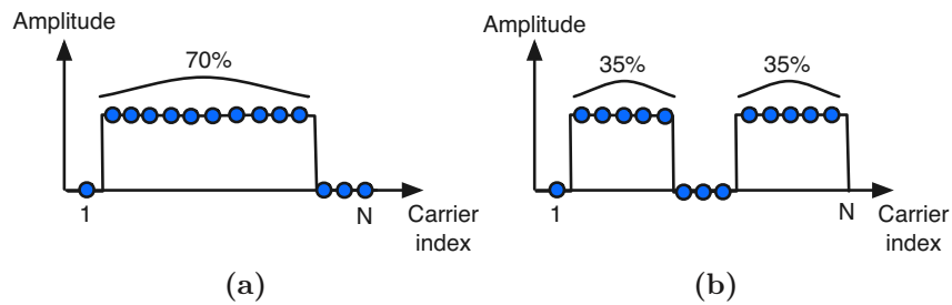
FIGURE 6.4 Gabarits spectraux étudiés
