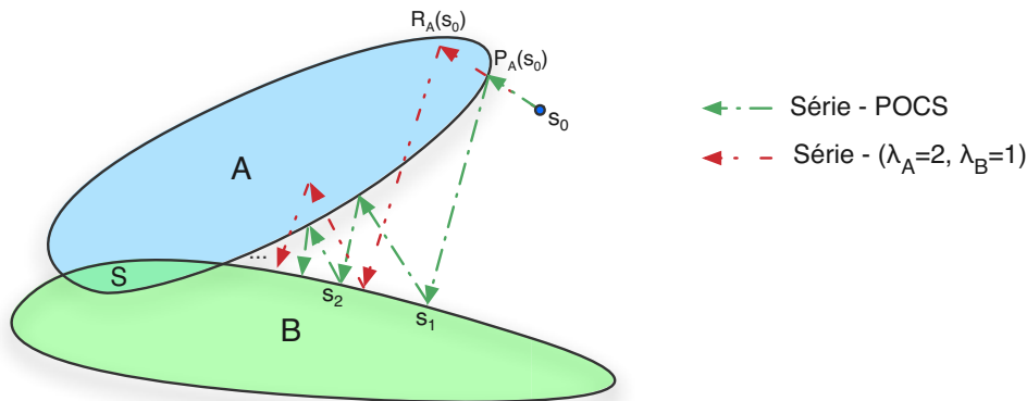
FIGURE 5.4 Algorithmes séries : POCS ( \lambda_A=\lambda_B=1 ) et ( \lambda_A=2, \lambda_B=1 )
