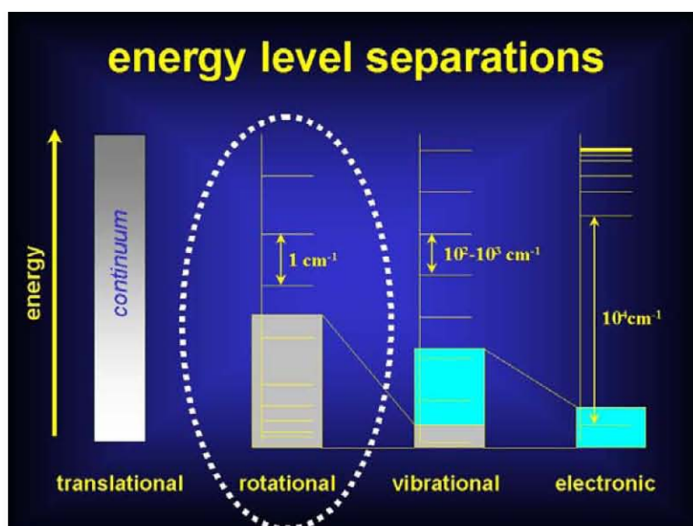
FIG. 2.3 Séparations typiques entre les niveaux électroniques, vibrationnels et rotationnels d'une molécule ( http://www.achem.ic.ac.uk/demello/teaching/l3/index.htm )
